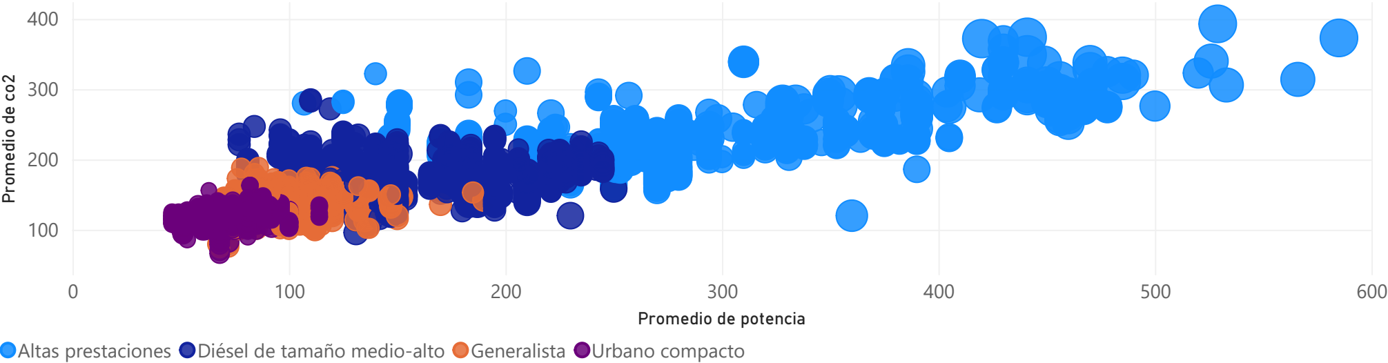
Potencia frente a emisiones · muestra de 60.000 vehículos
