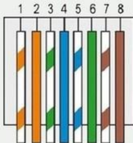
T568B
