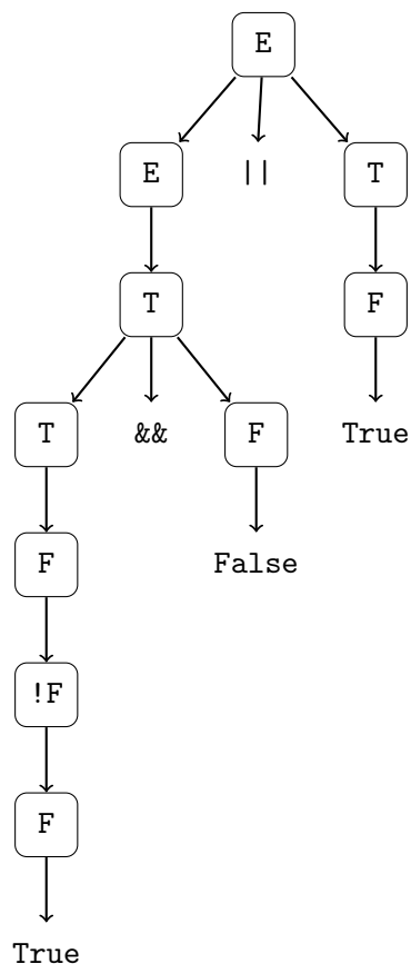
FIGURE 1 – Arbre d'analyse syntaxique de !True && False || True
