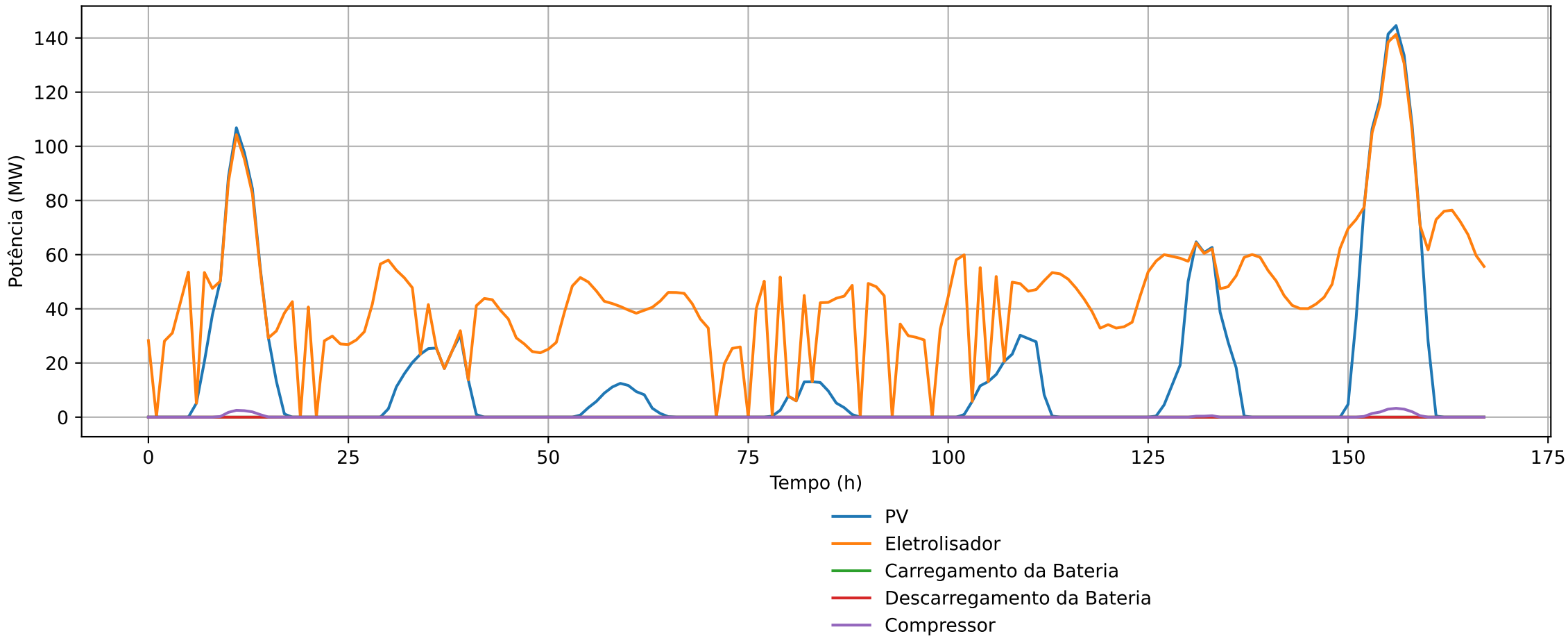
Potência por Cenário - p5
