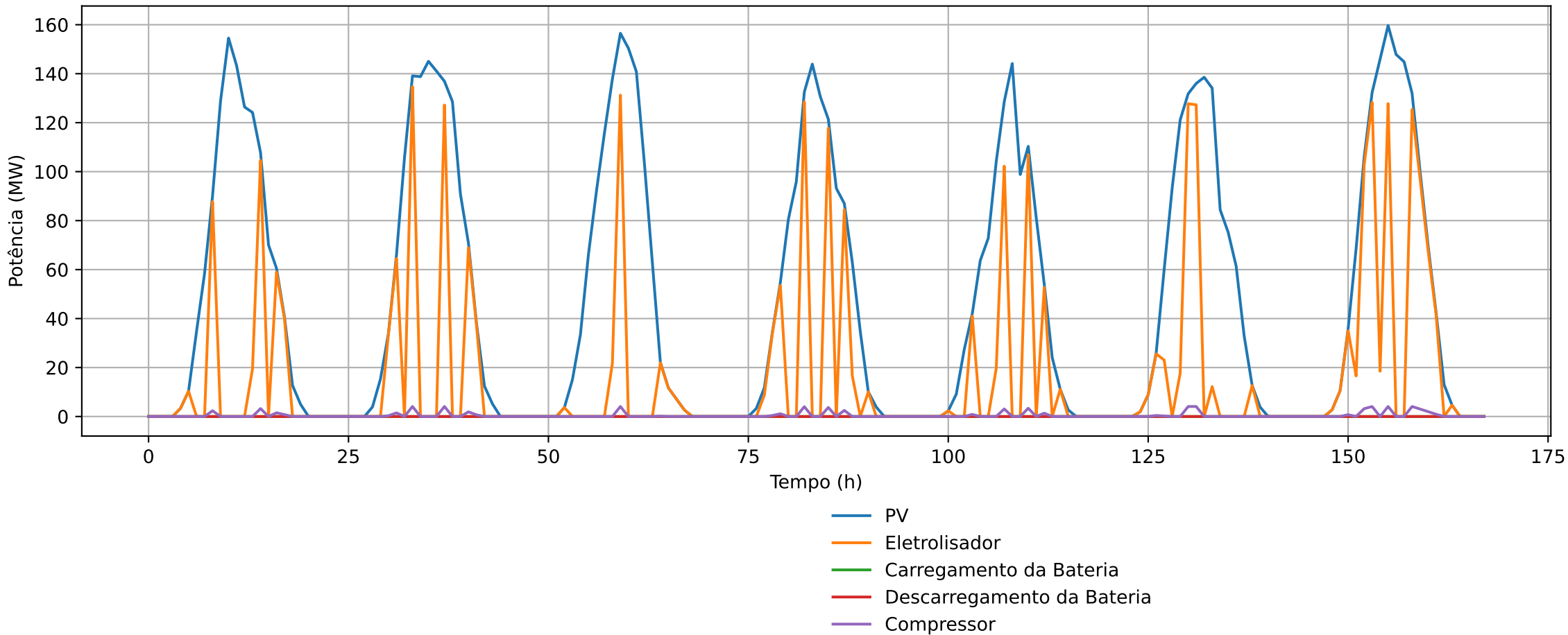
Potência por Cenário - p1
