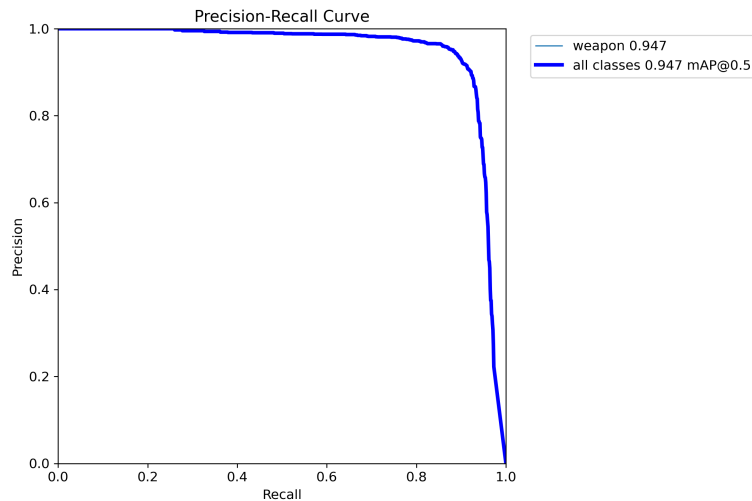
Figura 4.8: Curba precizie-sensibilitate ( precision-recall ) obținută de detectorul de arme pe setul de validare. Aria de sub curbă reflectă valoarea mAP@0,5 = 0,947. Precizia rămâne cvasi-constantă, aproape de nivelul maxim, până la o sensibilitate de \approx 0,9 , demonstrând capacitatea sistemului de a identifica majoritatea țintelor cu o incidență minimă a alarmelor false.
