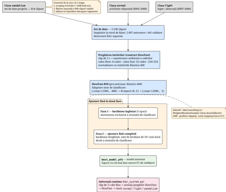
Figura 5.9: Procesul modului de recunoaștere a acțiunilor umane. Setul de date este alcătuit din trei clase: normal , fight și vandalism . Clipurile sunt împărțite la nivel de fișier în antrenare și validare, iar fiecare clip este transformat, conform contractului SlowFast , într-o pereche de intrări Slow/Fast . Modelul SlowFast R50 pre-antrenat pe Kinetics-400 primește un strat nou de clasificare cu trei ieșiri și este ajustat fin în două faze. Modelul rezultat ( best_model.pth ) este apoi folosit la inferență în aplicație, unde clasifică, prin aceeași pregătire a intrărilor, clipuri de două secunde.
