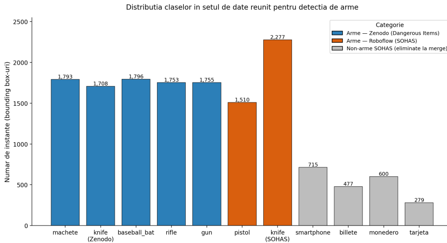
Figura 5.6: Distribuția casetelor de încadrare ( bounding boxes ) pe clasele originale ale celor două seturi de date, anterior remapării la categoria unică weapon . Cromatica indică proveniența și tipologia datelor: albastru pentru cele cinci clase de arme din setul Zenodo, portocaliu pentru clasele de arme reținute din SOHAS ( pistol și knife ), respectiv gri pentru clasele non-armă din SOHAS (excluse la unificare și reutilizate drept exemple negative). Categoria knife , comună ambelor surse, este reprezentată distinct. Valorile afișate deasupra barelor indică volumul total de adnotări, cumulat pentru partițiile de antrenare, validare și testare.
