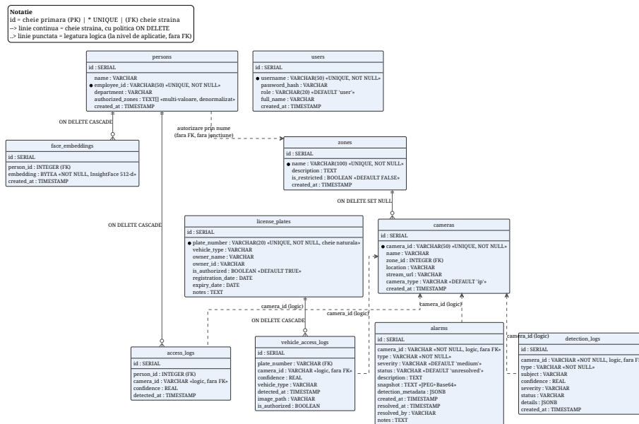
Figura 4.8: Diagrama entitate-relație (ERD) a schemei PostgreSQL facial_recognition , cu cele zece tabele implementate în database_manager.py . Cheile primare ( id ) sunt subliniate, iar cele cinci constrângeri UNIQUE sunt marcate cu asterisc. Liniile punctate evidențiază legăturile logice neimpuse prin FK: cele patru câmpuri camera_id către cameras și relația persoană-zonă, denormalizată ca atribut multi-valoare authorized_zones TEXT[] pe persons (nu ca entitate asociativă). Tabelul users este independent.
