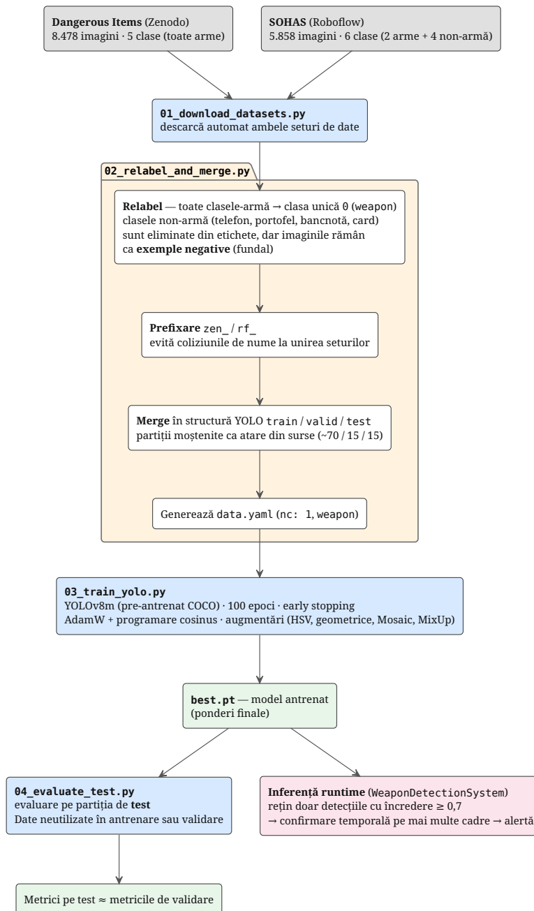
Figura 5.5: Fluxul de date și antrenare a detectorului de arme. Cele patru scripturi execută secvențial: (1) descărcarea seturilor Zenodo și Roboflow; (2) unificarea lor (remapare pe o clasă, reținerea exemplilor negative și formatare YOLO); (3) antrenarea modelului YOLOv8m ( best.pt ); (4) evaluarea pe datele de test. Ponderile validate sunt ulterior integrate în aplicația de supraveghere.
