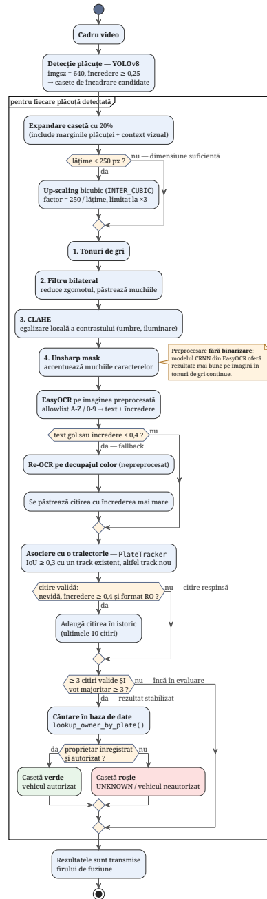
Figura 5.3: Fluxul de procesare al modului de recunoaștere a plăcuțelor. Fiecare plăcuță detectată de YOLOv8 este decupată cu o margine de context, mărită dacă este prea mică și supusă unui lanț de patru operații de preprocesare. Doar după consensul pe minimum trei cadre se interoghează baza de date și se decide autorizarea (casetă verde) sau respingerea (casetă roșie).
