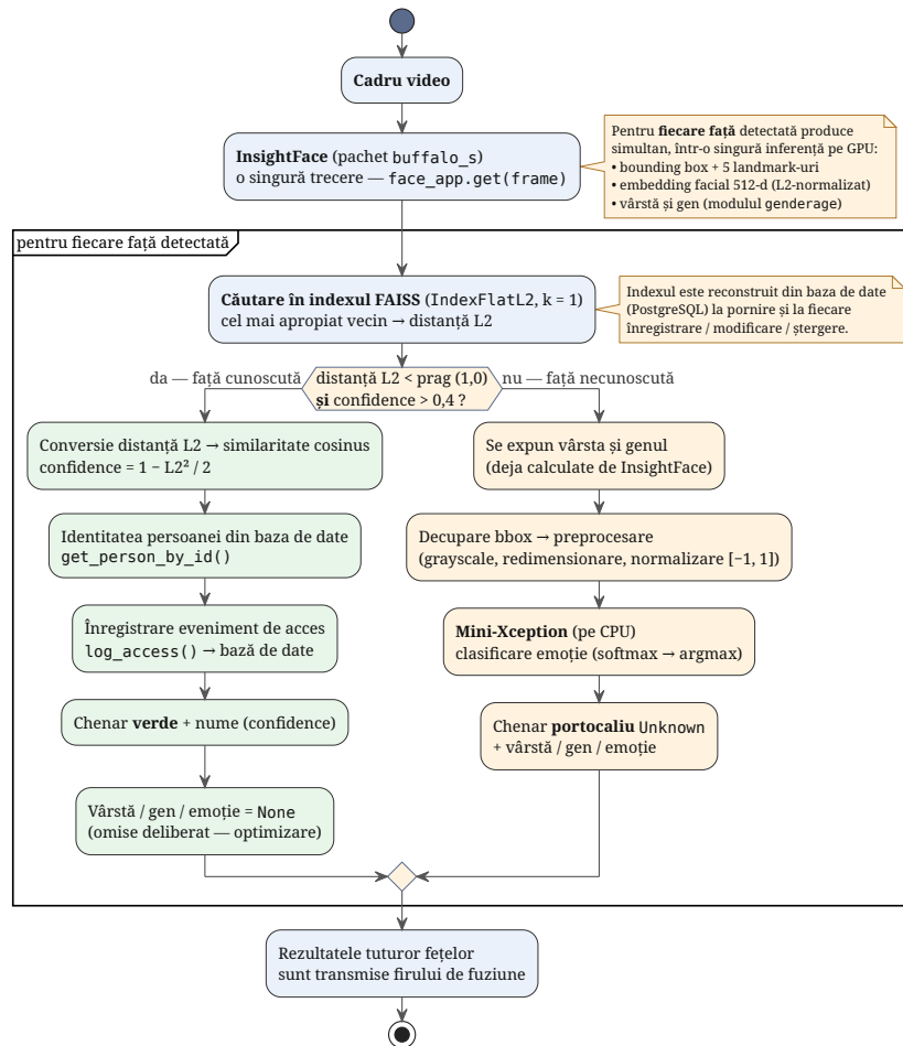
Figura 5.2: Fluxul de procesare al modulului de recunoaștere facială. Fiecare cadru este analizat de InsightFace într-o singură trecere, care produce simultan, pentru toate fețele, caseta de încadrare, embedding-ul de 512 dimensiuni și estimările demografice. Pentru fiecare față, embedding-ul este căutat în indexul FAISS, iar identitatea se stabilește pe baza unui prag dublu (distanță L_2 < 1,0 și încredere > 0,4 ). Fețele cunoscute (ramura verde) sunt jurnalizate ca evenimente de acces, iar atributele demografice sunt omise deliberat; fețele necunoscute (ramura portocalie) sunt caracterizate demografic, iar emoția este clasificată suplimentar de rețeaua Mini-Xception pe CPU. Indexul FAISS este reconstruit determinist din baza de date.
