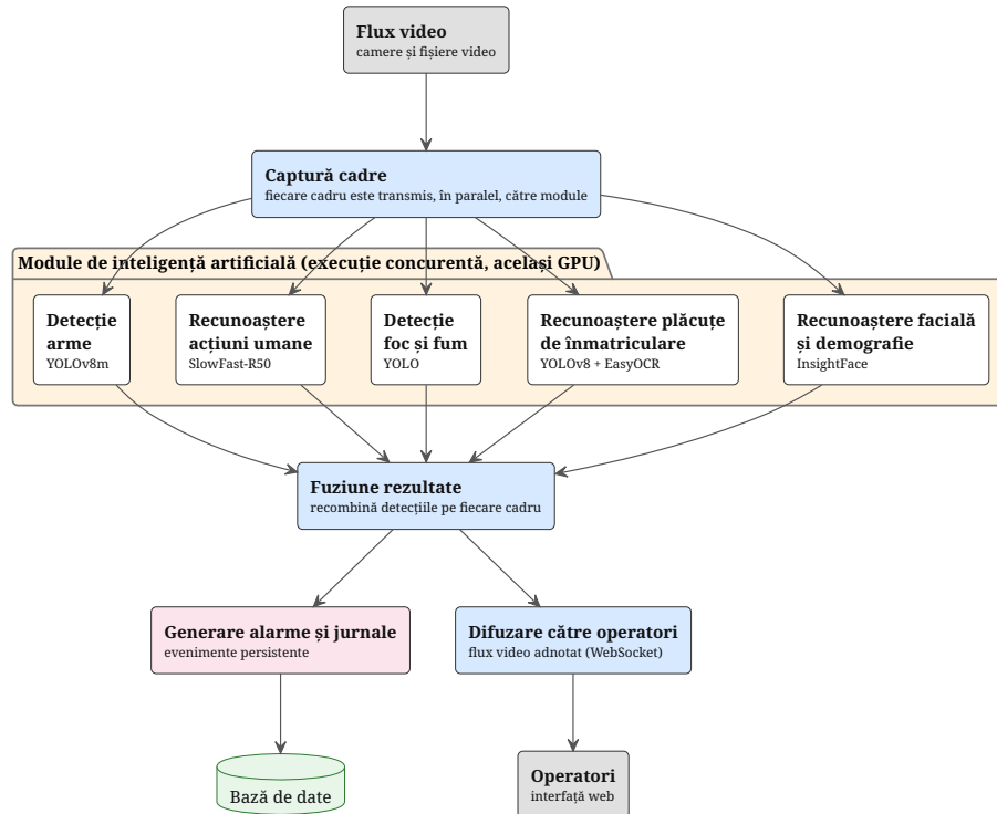
Figura 5.1: Imagine de ansamblu a fluxului de procesare al modulelor de inteligență artificială. Cadrele capturate din fluxul video sunt transmise, în paralel, către cele cinci module de inteligență artificială; sub fiecare modul este indicat modelul (sau biblioteca) pe care se bazează. Rezultatele converg în etapa de fuziune, care le recombina pe fiecare cadru, generează alarmele și jurnalele și difuzează cadrul adnotat către operatori. Pentru claritate, diagrama rămâne la nivel de ansamblu; detalierea firelor de execuție, a cozilor și a mecanismului de fuziune se găsește în Figura 4.6 și în Secțiunea 5.8.
