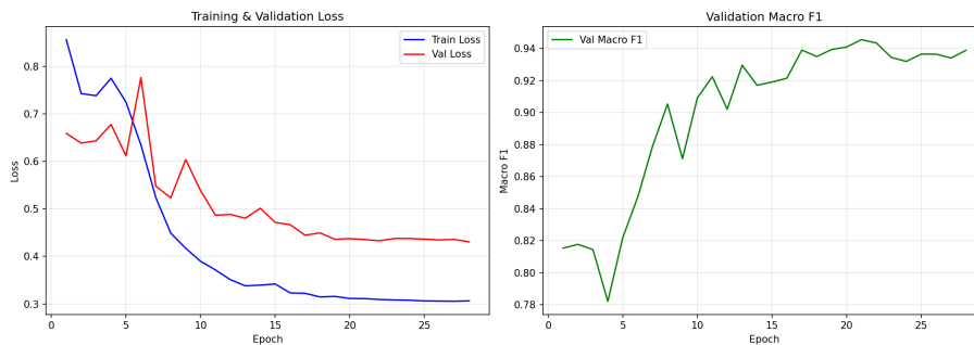
Figura 5.10: Evoluția antrenării modelului de recunoaștere a acțiunilor pe durata a 28 de epoci. Stânga: funcția de cost de antrenare (albastru) și de validare (roșu). Dreapta: scorul macro-F1 obținut pe setul de validare. Perturbarea din jurul epocilor 4–6 corespunde deblocării parametrilor rețelei de bază (tranziția de la ponderi fixe în epocile 1–5 la optimizare globală începând cu epoca 6). Ponderile optime s-au obținut la epoca 21, mecanismul de oprire timpurie ( early stopping ) declanșându-se la epoca 28.
