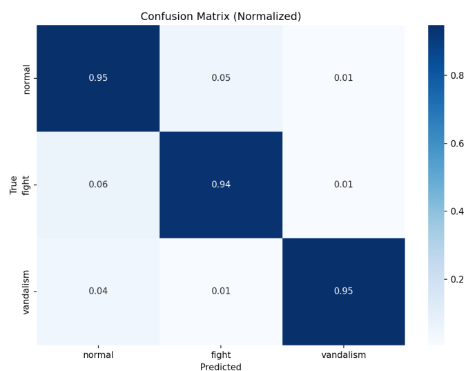
Figura 5.11: Matricea de confuzie normalizată a modelului de recunoaștere a acțiunilor, evaluată pe partiția de validare. Liniile indică apartenența reală la clasă ( ground truth ), în timp ce coloanele reprezintă predicțiile modelului, valorile fiind normalizate pe fiecare linie. Dominanța valorilor de pe diagonala principală confirmă acuratețea ridicată a clasificării, erorile reziduale manifestându-se cu precădere sub forma unor confuzii între clasele normal și fight .
