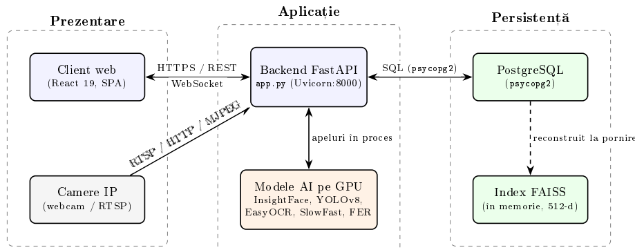
Figura 4.3: Diagramă bloc de ansamblu a sistemului, organizată pe cele trei straturi logice (Prezentare, Aplicație, Persistentă) și protocolele de comunicare dintre componente: HTTPS/REST și WebSocket între client și backend, RTSP/HTTP/MJPEG pentru fluxurile camerelor, apeluri în proces către modelele AI de pe GPU și acces SQL la PostgreSQL prin driver-ul psycopg2 . Indexul FAISS este menținut în memoria backend-ului și reconstruit din PostgreSQL la pornire.
