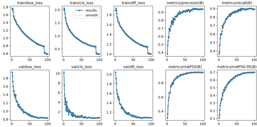
Figura 5.7: Curbele de antrenare ale detectorului de arme pe parcursul celor 100 de epoci. Rândul superior: componentele funcției de cost pe partiția de antrenare ( box_loss , cls_loss , dfl_loss ), precizia și sensibilitatea. Rândul inferior: aceleași componente de cost pe partiția de validare, împreună cu metricile mAP@0,5 și mAP@0,5:0,95. Punctele reprezintă valorile per epocă, iar linia punctată roșie varianta netezită. Scăderea bruscă a costului de antrenare în jurul epocii 90 corespunde dezactivării augmentării mosaic în ultimele zece epoci.
