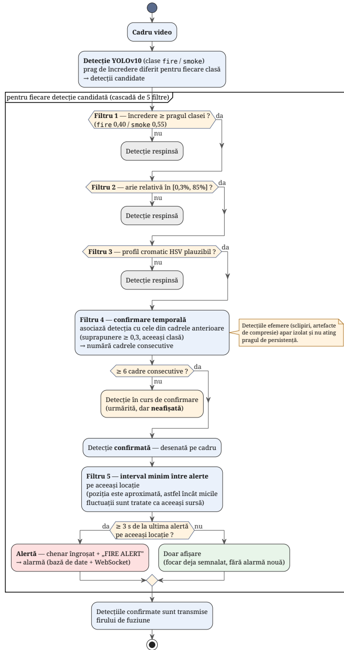
Figura 5.4: Cascada de filtrare foc/fum. Detecțiile YOLOv10 parcurg cinci etape: încredere, dimensiune, analiză HSV, agregare temporală IoU și cooldown . Rezultatele sunt progresiv respinse (gri), în așteptare (portocaliu), confirmate vizual (verde) sau marcate ca alertă (roșu). Indicatorii confirmed și alert separă starea validată de evenimentul declanșat.
