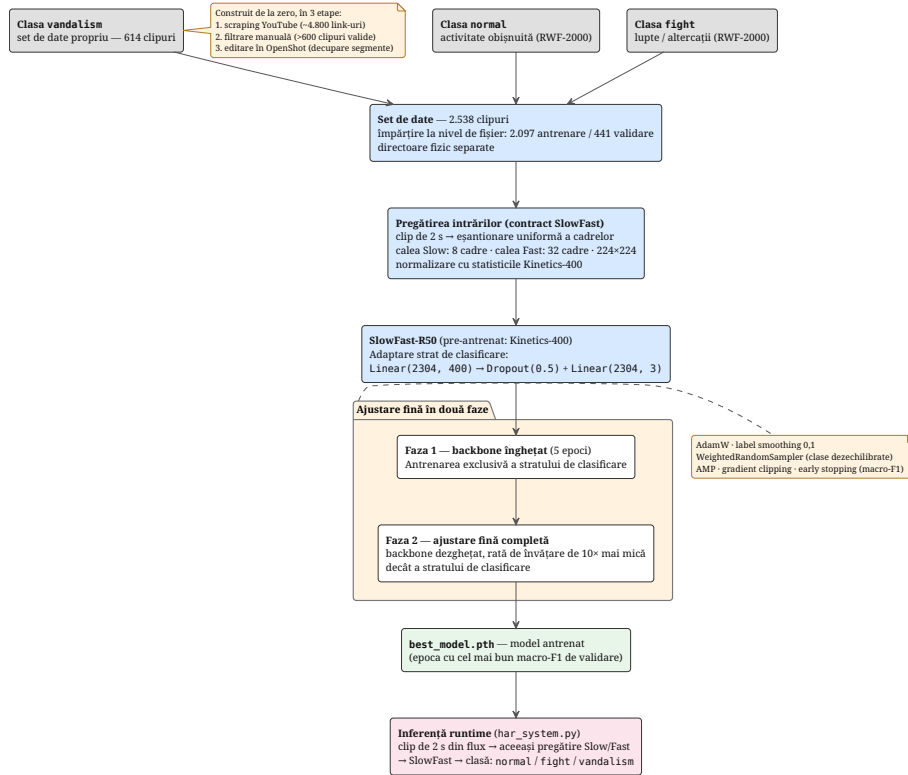
Figura 5.9: Procesul modulului de recunoaștere a acțiunilor umane. Setul de date este alcătuit din trei clase: normal , fight și vandalism . Clipurile sunt împărțite la nivel de fișier în antrenare și validare, iar fiecare clip este transformat, conform contractului SlowFast, într-o pereche de intrări Slow/Fast. Modelul SlowFast R50 pre-antrenat pe Kinetics-400 primește un strat nou de clasificare cu trei ieșiri și este ajustat fin în două faze. Modelul rezultat ( best_model.pth ) este apoi folosit la inferență în aplicație, unde clasifică, prin aceeași pregătire a intrărilor, clipuri de două secunde.
