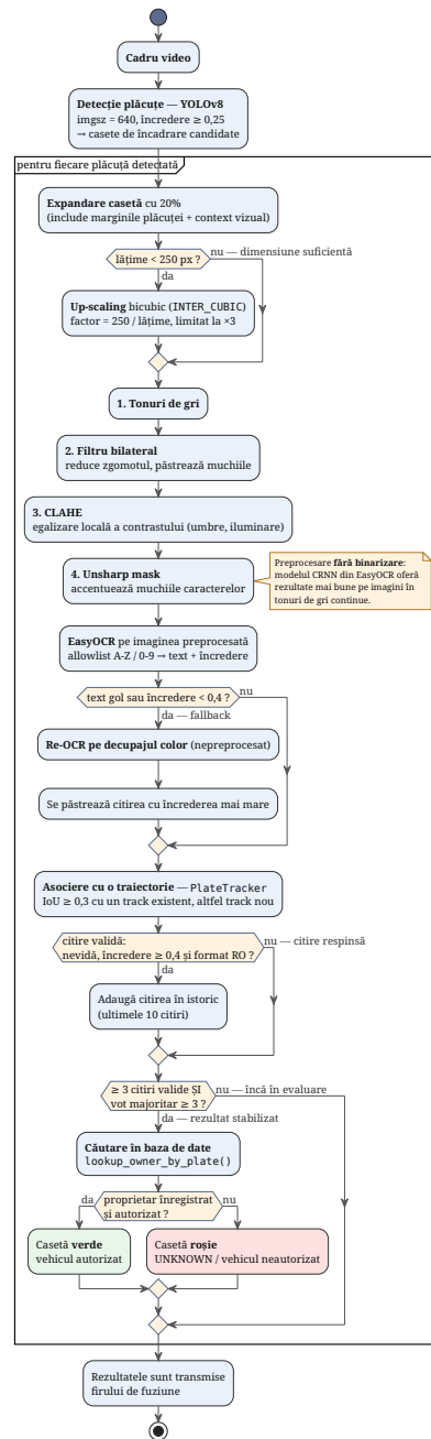
Figura 5.3: Fluxul de procesare al modulului de recunoaștere a plăcuțelor. Fiecare plăcuță detectată de YOLOv8 este decupată cu o margine de context, mărită dacă este prea mică și supusă unui lanț de patru operații de preprocesare. Doar după consensul pe minimum trei cadre se interoghează baza de date și se decide autorizarea (casetă verde) sau respingerea (casetă roșie).
