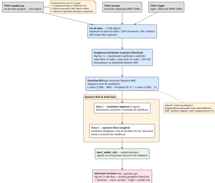
Figura 5.7: Procesul modulului de recunoaștere a acțiunilor umane. Setul de date este alcătuit din trei clase: normal , fight și vandalism . Clipurile sunt împărțite la nivel de fișier în antrenare și validare, iar fiecare clip este transformat, conform contractului SlowFast, într-o pereche de intrări Slow/Fast. Modelul SlowFast R50 pre-antrenat pe Kinetics-400 primește un strat nou de clasificare cu trei ieșiri și este ajustat fin în două faze. Modelul rezultat ( best_model.pth ) este apoi folosit la inferență în aplicație, unde clasifică, prin aceeași pregătire a intrărilor, clipuri de două secunde.
