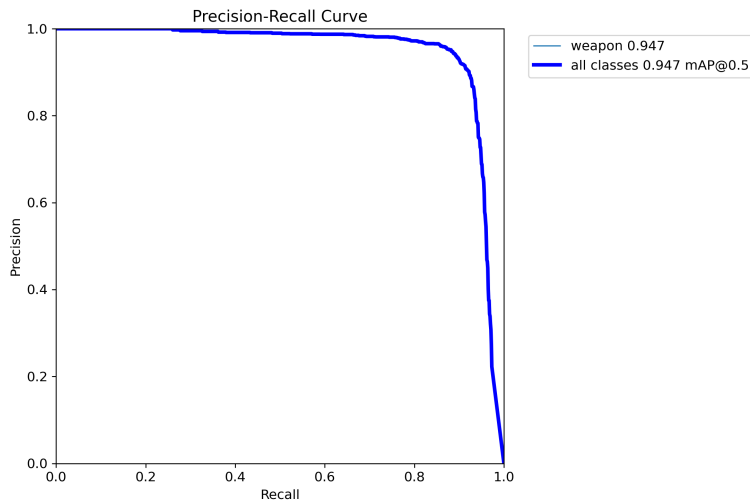
Figura 5.8: Curba precizie-sensibilitate ( precision-recall ) obținută de detectorul de arme pe setul de validare. Aria de sub curbă reflectă valoarea mAP@0,5 = 0,947. Precizia rămâne cvasi-constantă, aproape de nivelul maxim, până la o sensibilitate de \approx 0,9 , demonstrând capacitatea sistemului de a identifica majoritatea țintelor cu o incidență minimă a alarmelor false.
