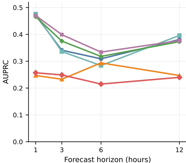
A. AUPRC
