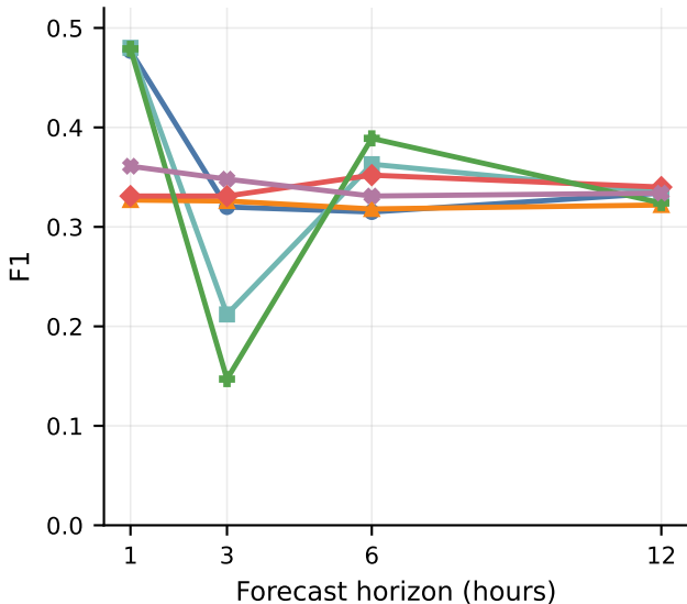
B. F1
