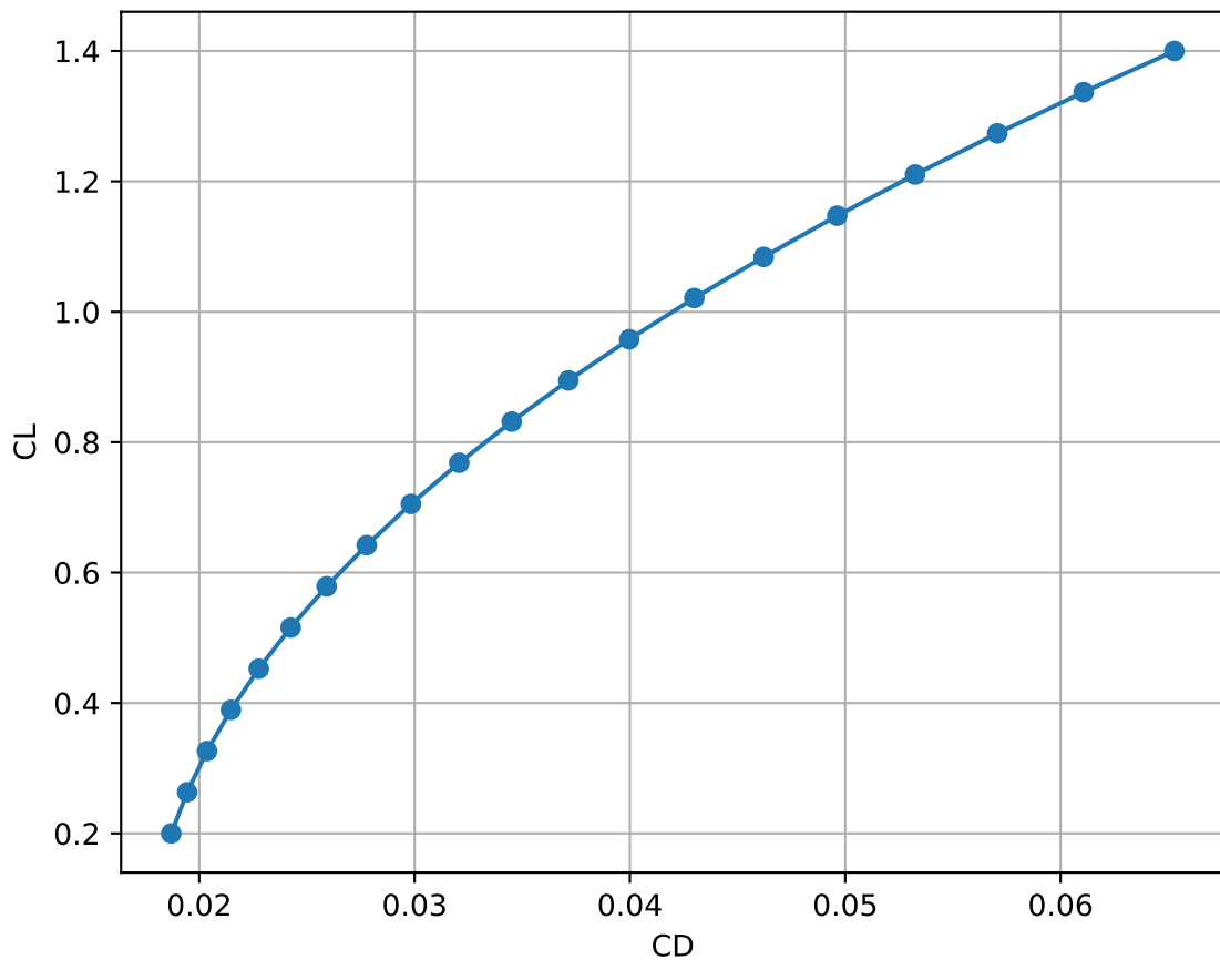
Polar de arrasto - Cruzeiro
