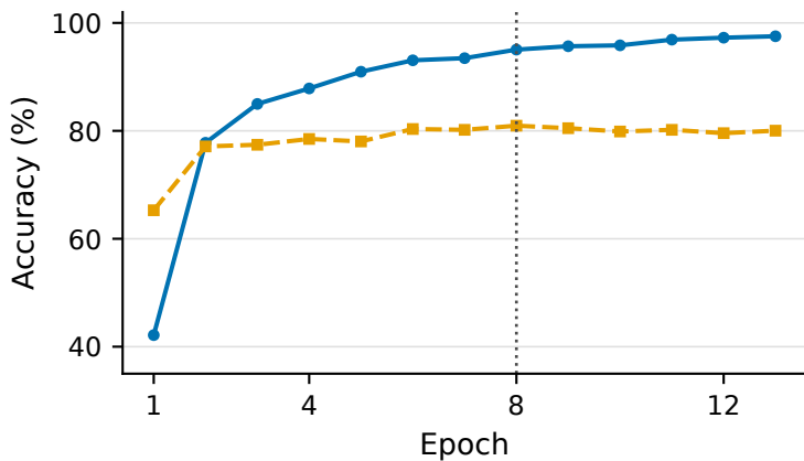
(c) R50-LP
