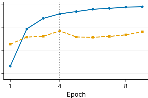
(d) R50-FT
