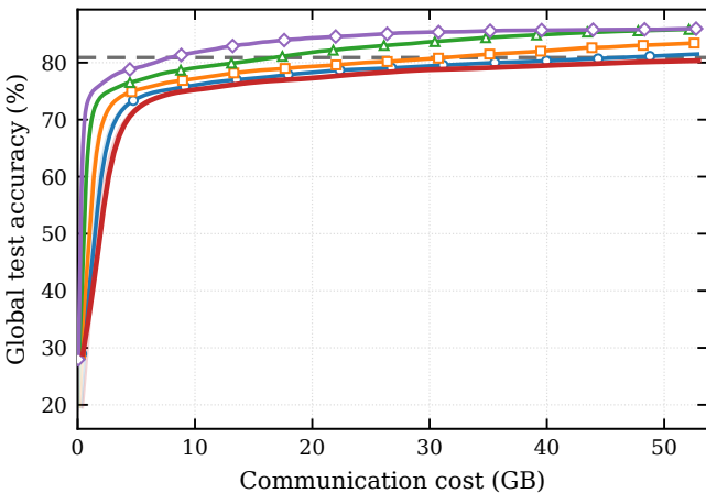
MNIST
