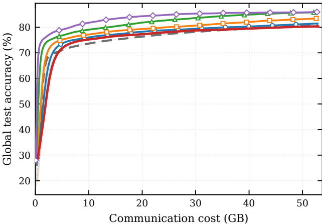
MNIST
