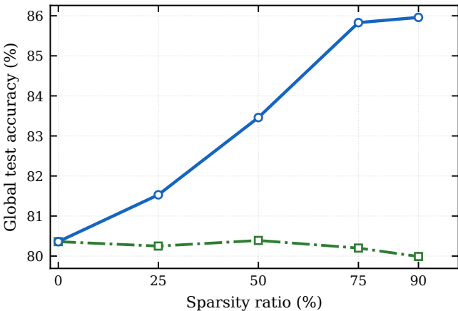
MNIST
