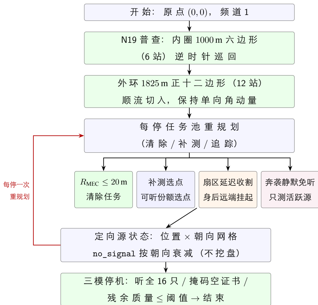
图 11 问题四算法整体流程 (N19 + 逆时针顺流 + 扇区延迟收割 + 奔袭静默免听)
