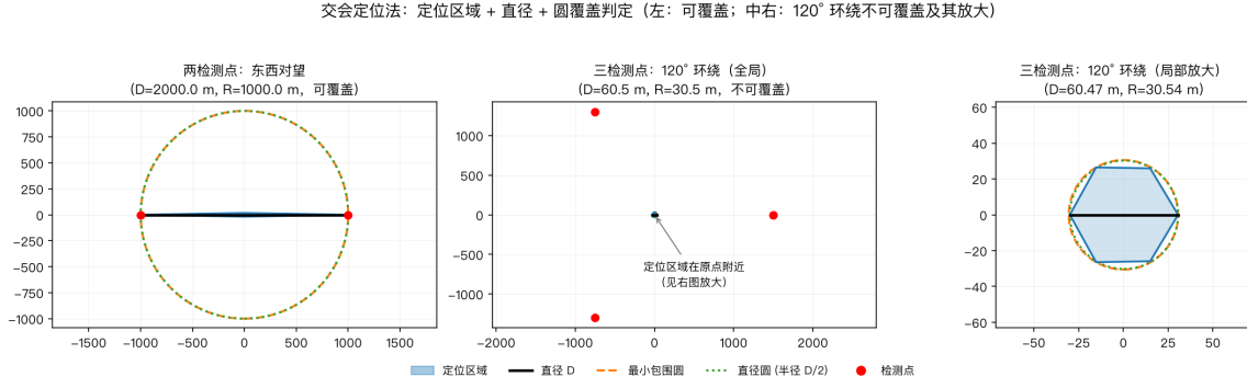
图 3 交会定位算例：定位区域、直径、最小包围圆与直径圆
