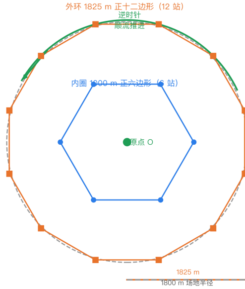
图 10 N19 超凸包普查站网（圆心 + 内圈 1000 m 六边形 + 外环 1825 m 正十二边形）
