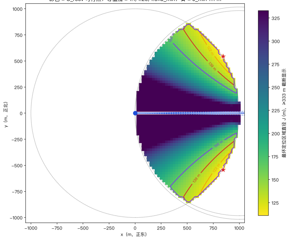
图 4 中心构型候选区域 (彩色为可行域最坏直径, 等值线为 1.1/1.25/1.5 \times J_{\min} , \star 为最优点)
