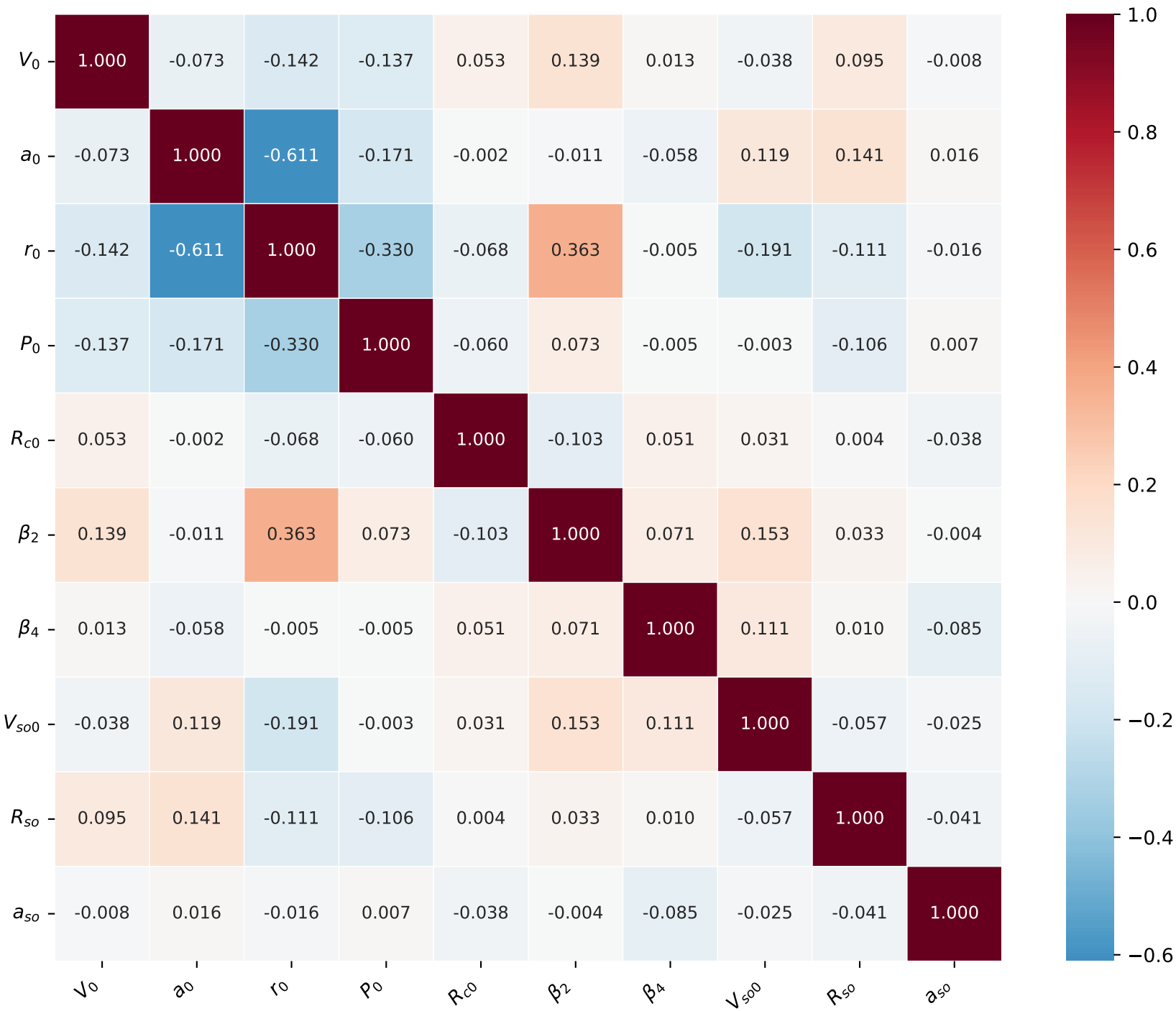
Posterior Correlation Matrix (145Tm)
