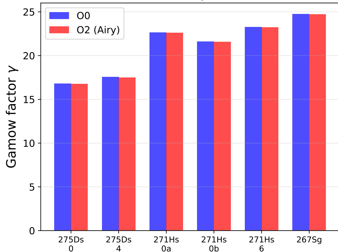
275 Ds decay chain
