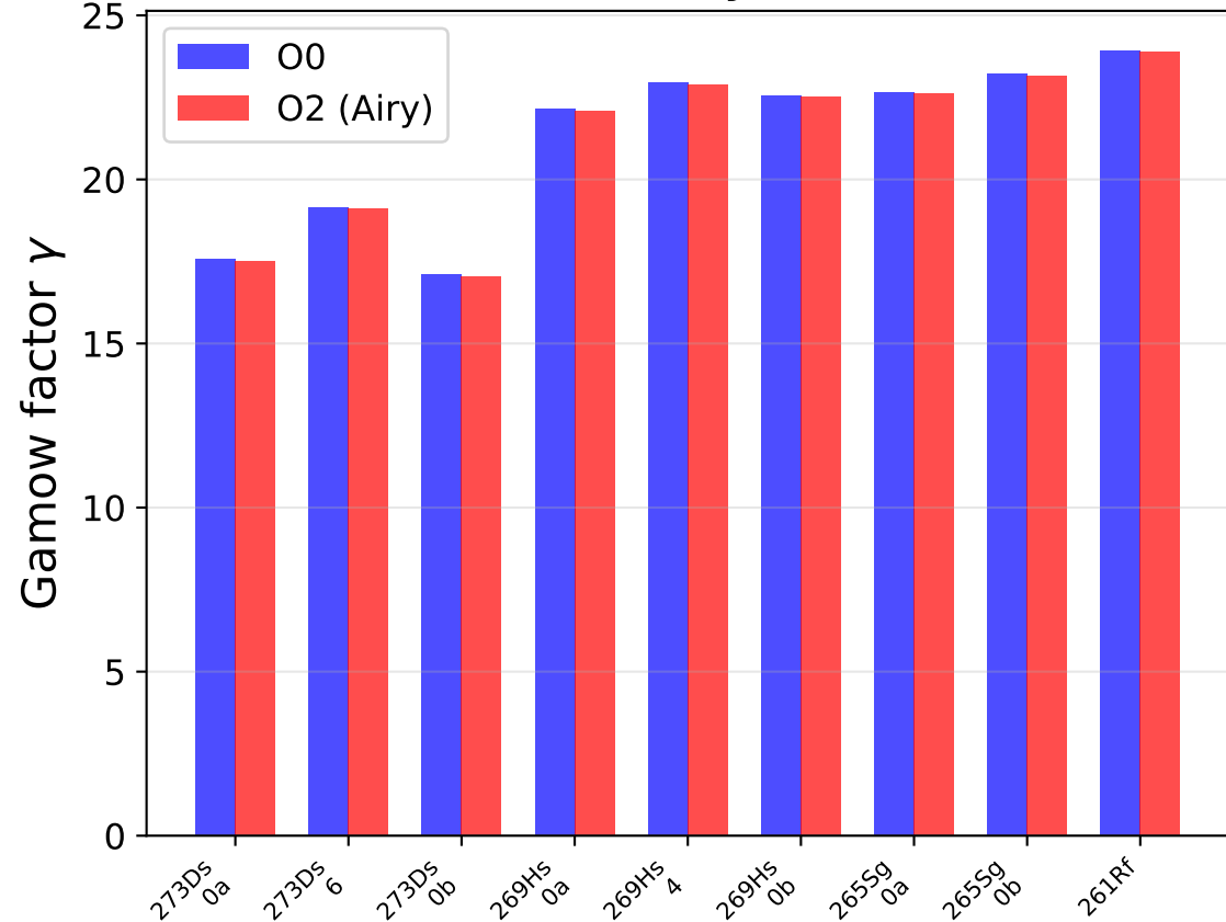
273 Ds decay chain
