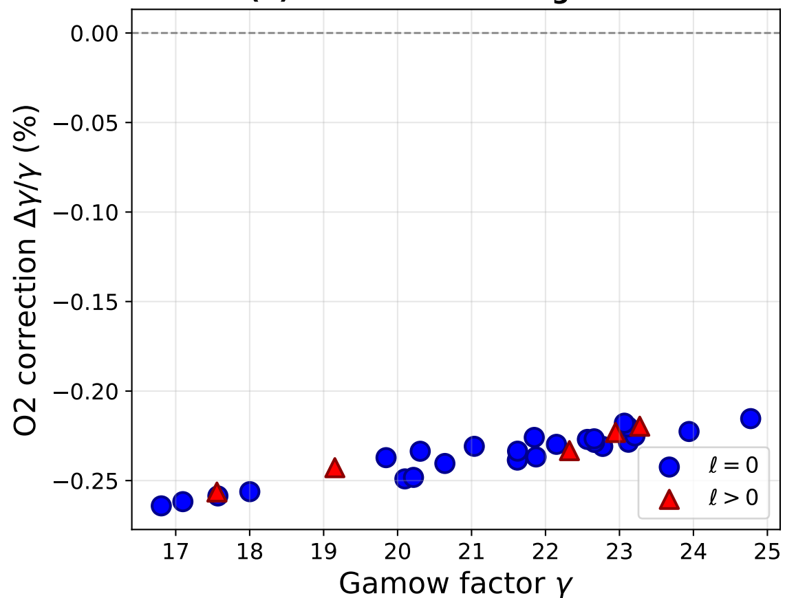
(b) O2 Correction Magnitude
