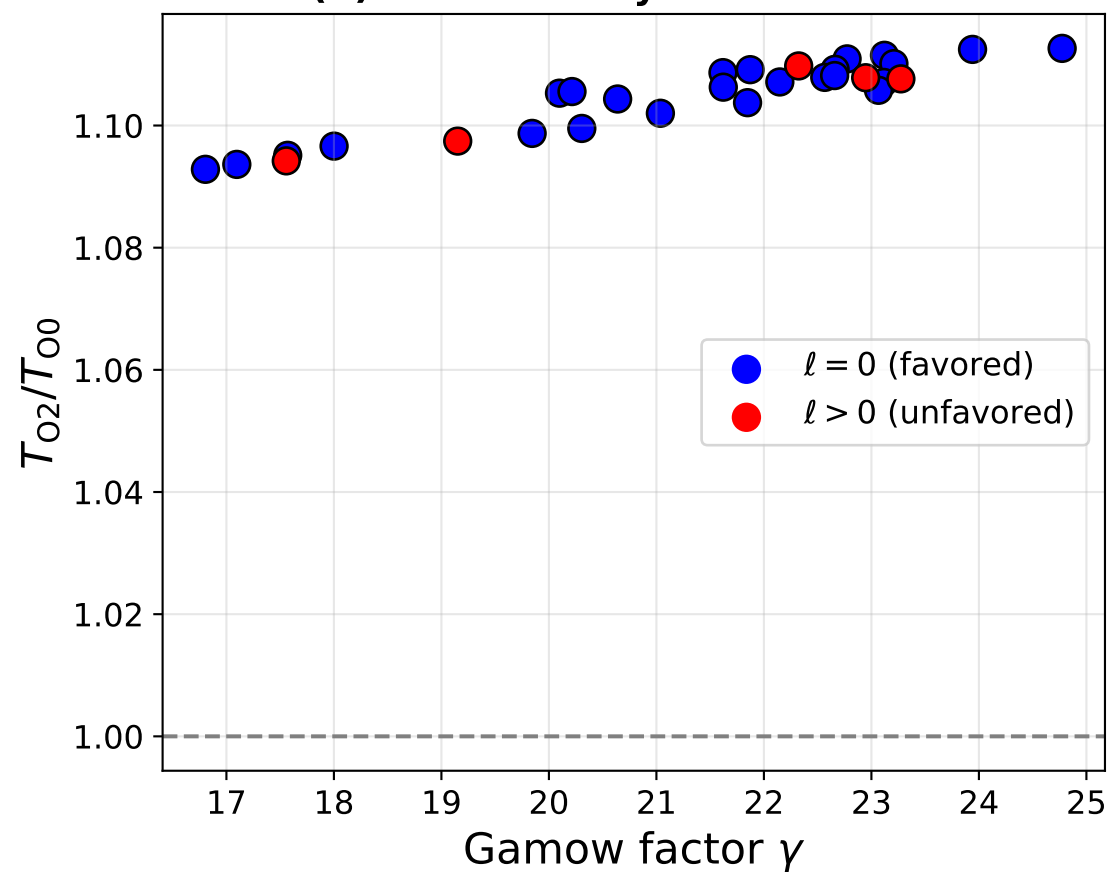
(d) Penetrability Enhancement
