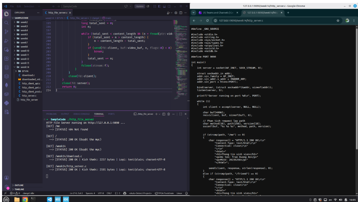
Hình 16 – File http_server.c
