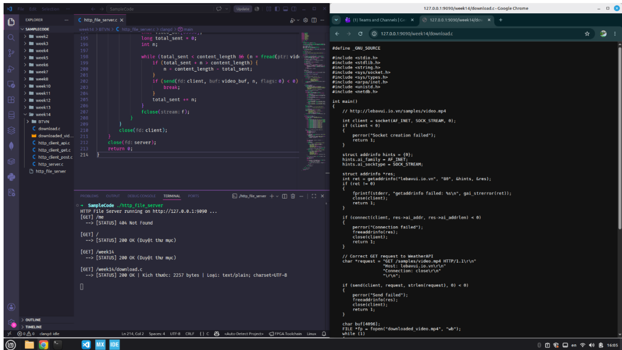
Hình 15 – File download.c
