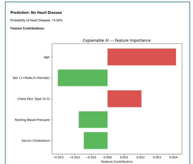
Fig. 3. SHAP OUTPUT 1
