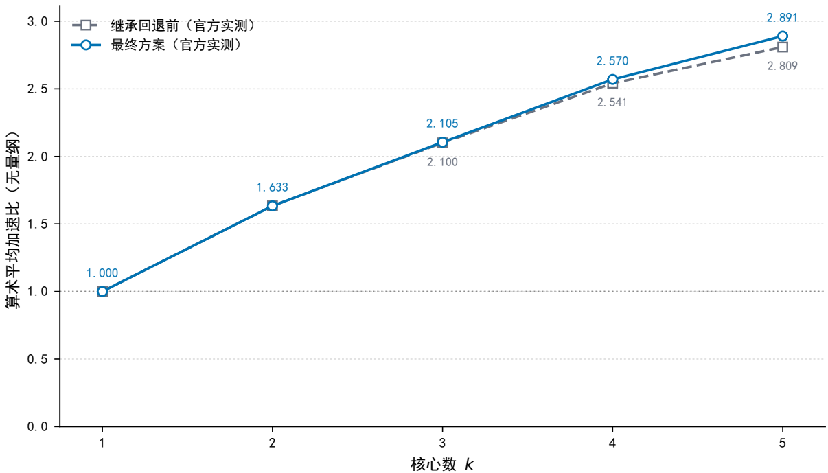
问题一：1~5 核平均加速比
