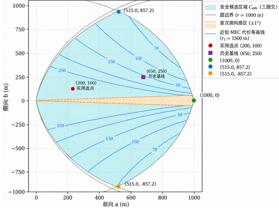
图3 保证接收的第二检测点候选区域及其等代价线
