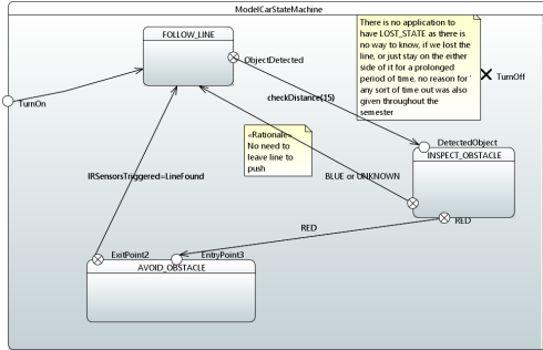
Fig. 17. ModelCarStateMachine
