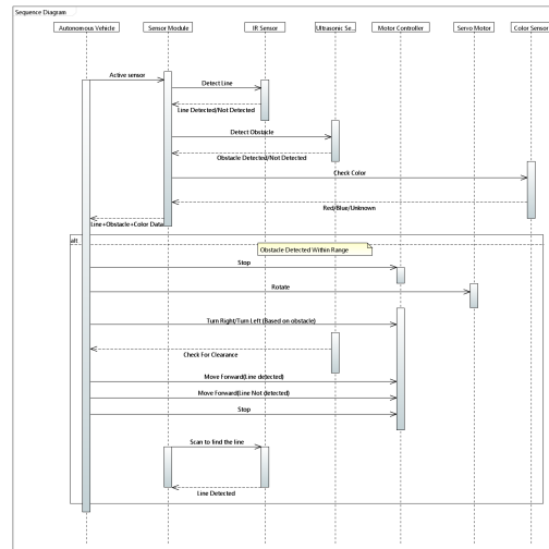
Fig. 16. SequenceDiagram
