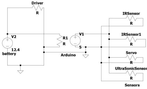
Fig. 13. Power Wiring
