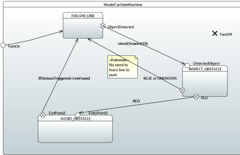
Fig. 17. ModelCarStateMachine
