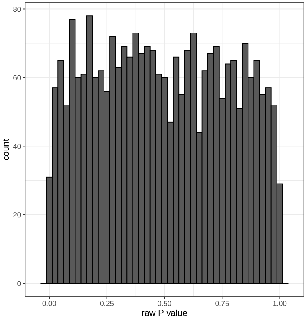
Training_CRE
