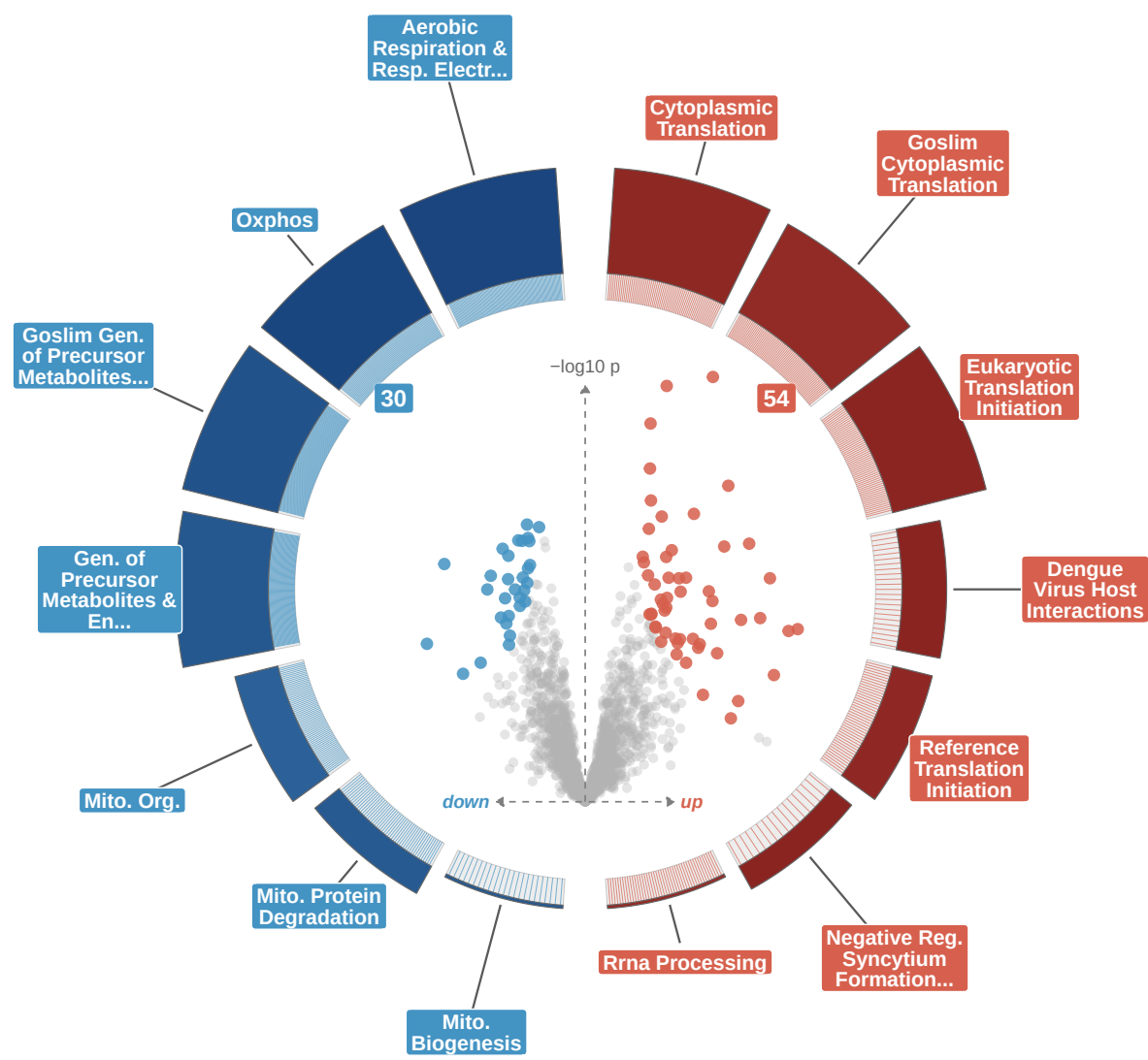
Acute_HR
