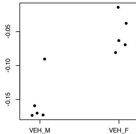
HALLMARK_PI3K_AKT_MTOR_SIGNALING AUC 0.00, p 0.008
