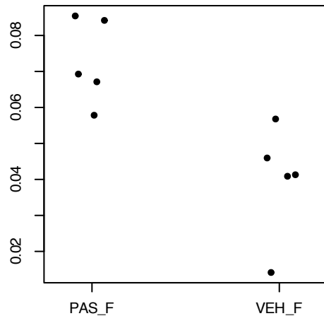
GOBP_INTRINSIC_APOPTOTIC_SI... AUC 1.00, p 0.008
