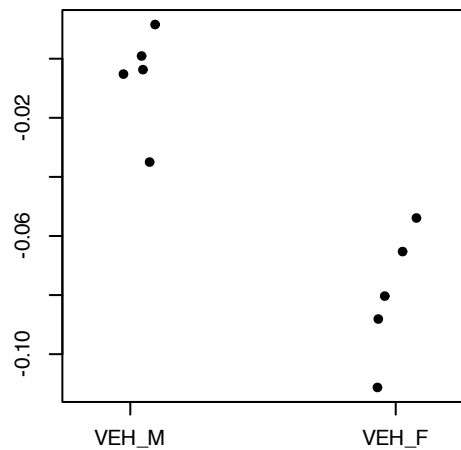
HALLMARK_DNA_REPAIR AUC 1.00, p 0.008
