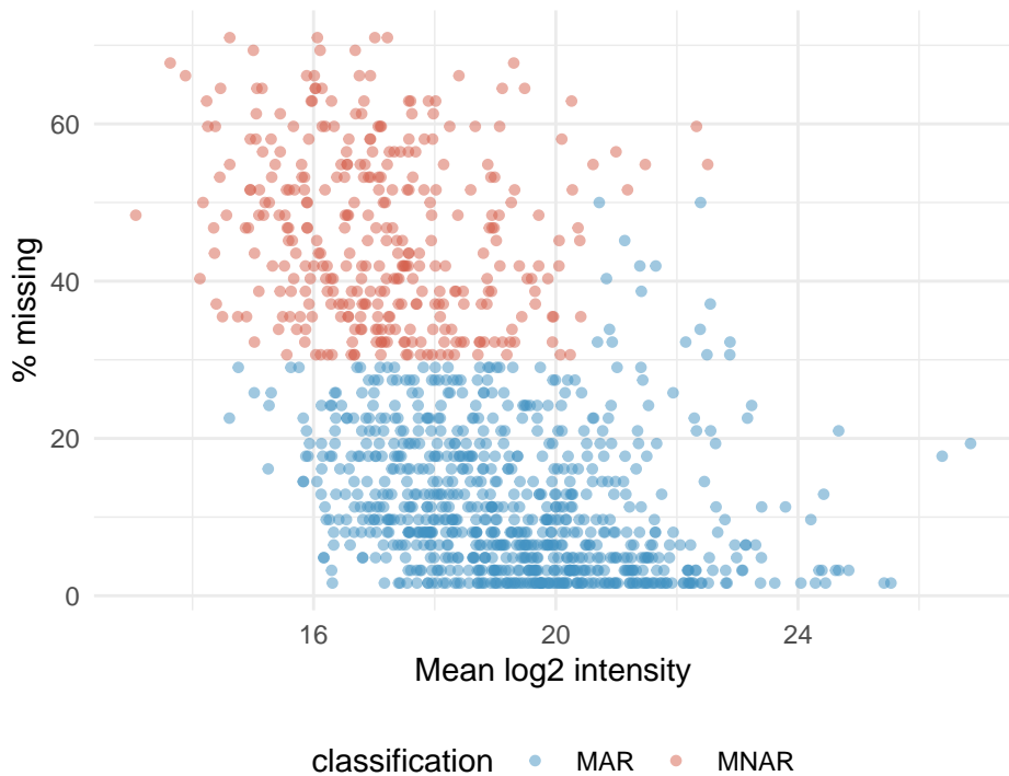
A: MAR vs MNAR
