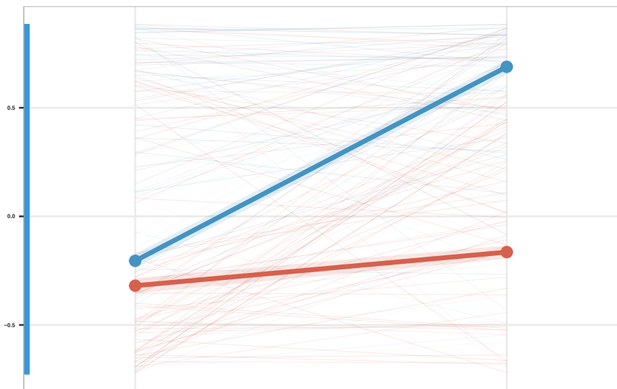
C3: OXPHOS (n = 530)
