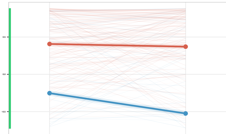
C4: Glycolysis (n = 565)
