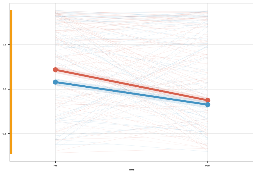
C4: Glycolysis (n = 565)
