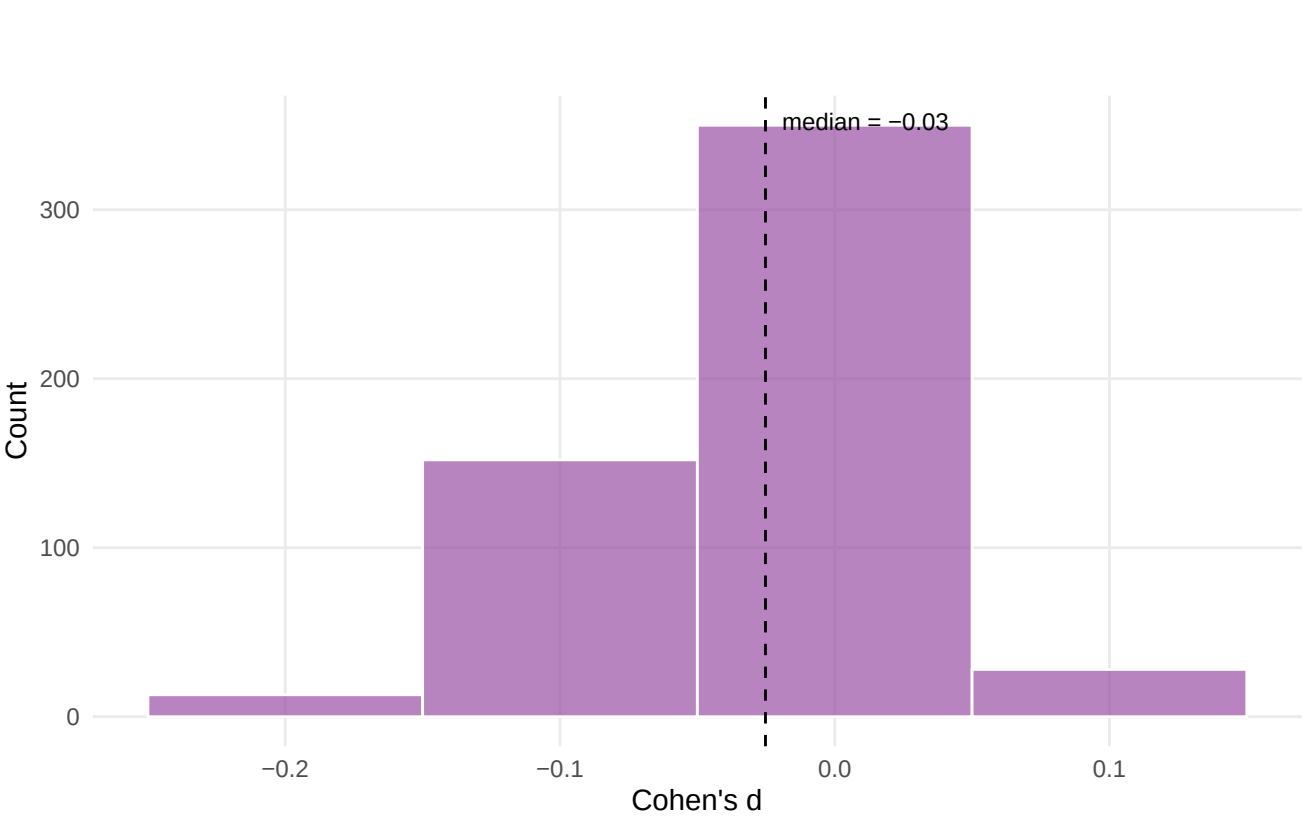
C. Imputation shift (MNAR)
