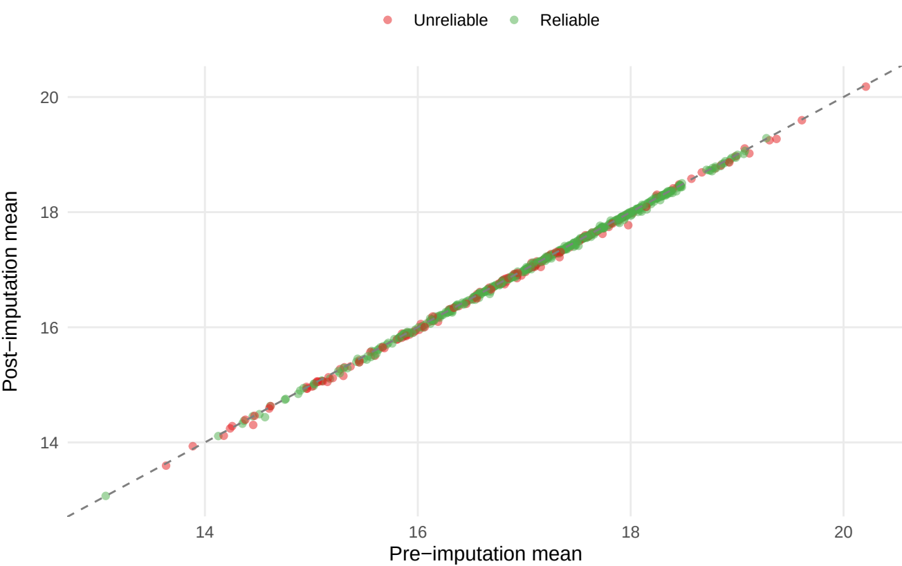
B. MNAR audit
