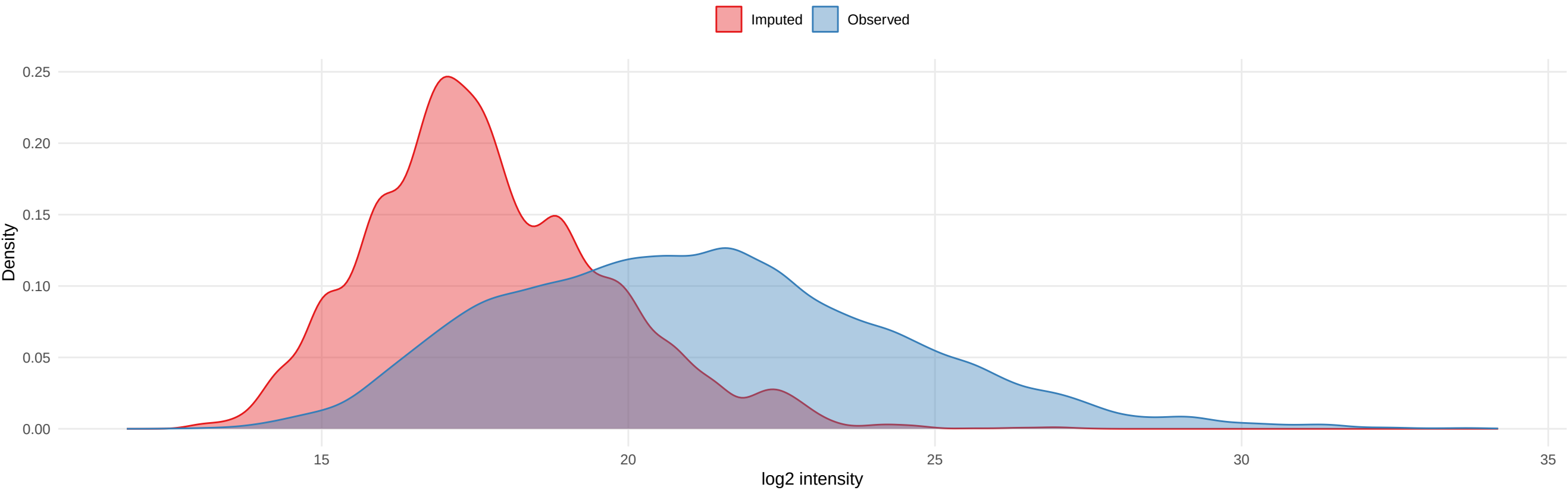
B. MNAR audit
