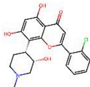
Alvocidib
