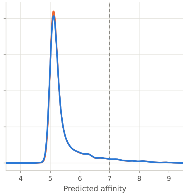
Prot2Drug
