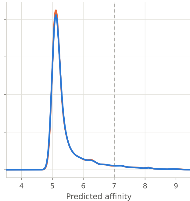
DeepDTAGen
