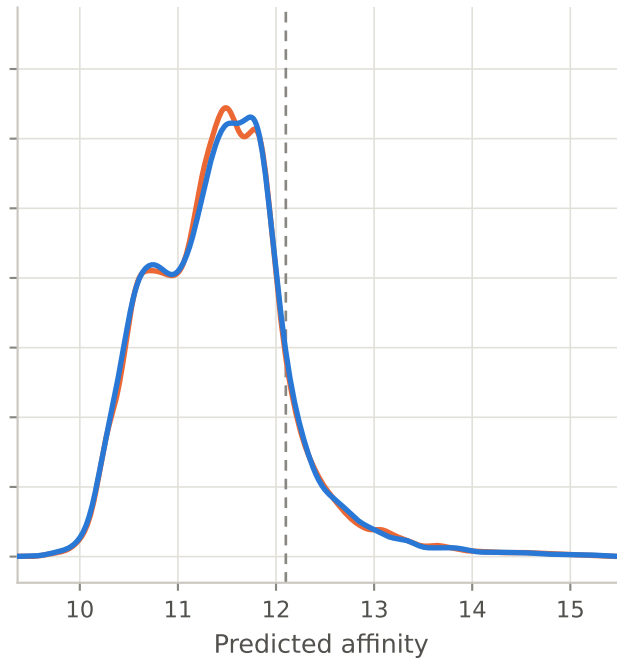
DeepDTAGen
