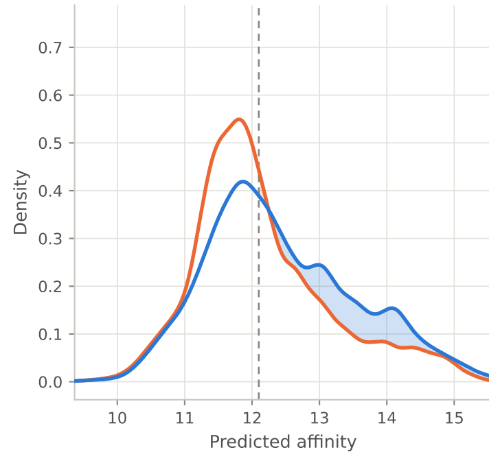
SelVAEGen
