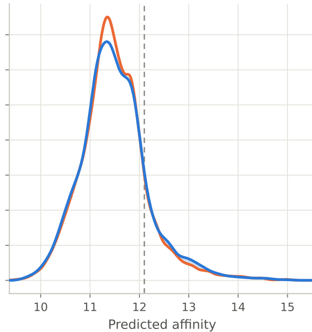
Prot2Drug
