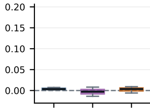
U(G_\omega, \tau)
