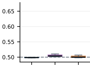
Dir. Cons.
