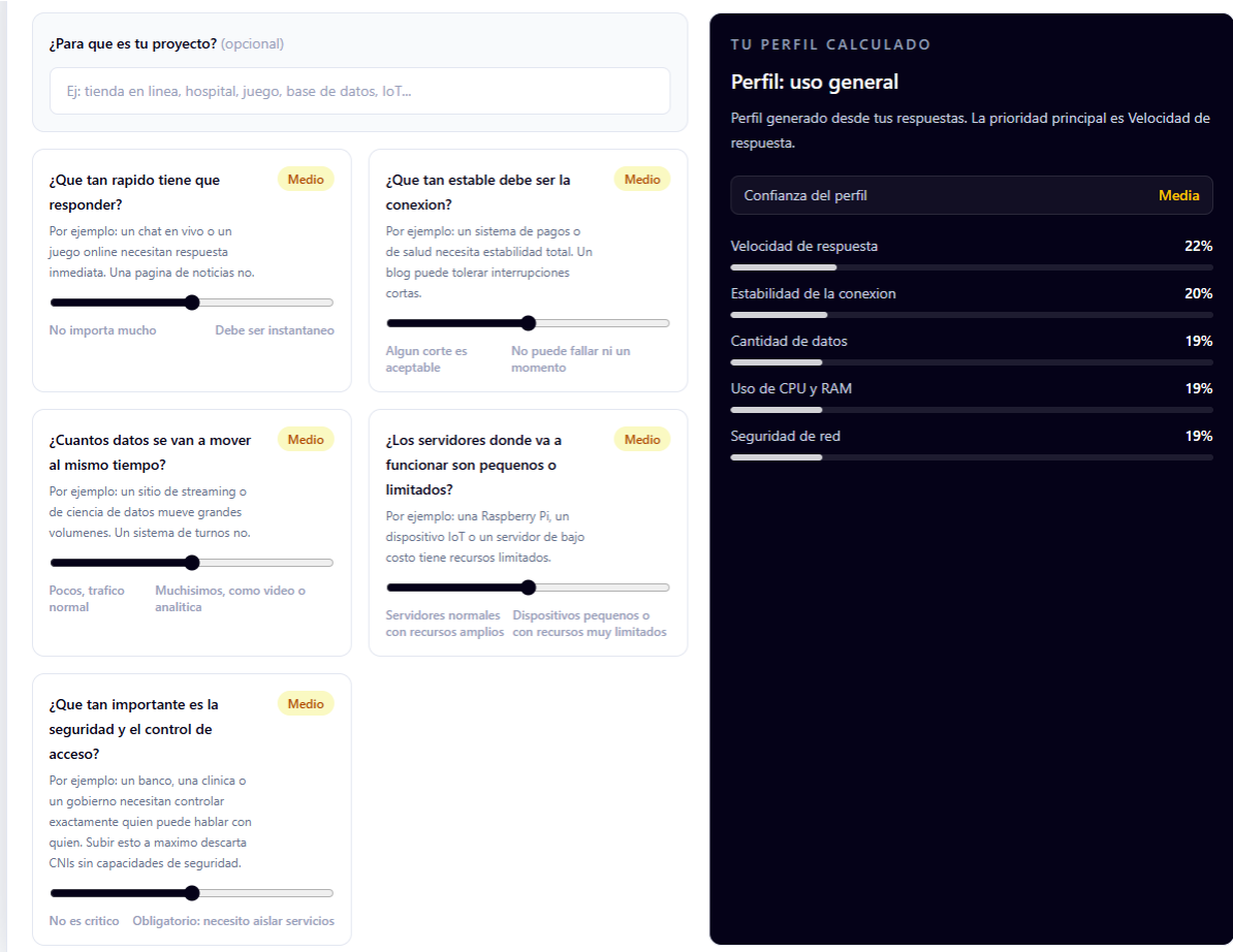
Figura A.4: Pantalla principal del recomendador SPA: GuidedProfileBuilder e indicador de fuente de datos activa.
