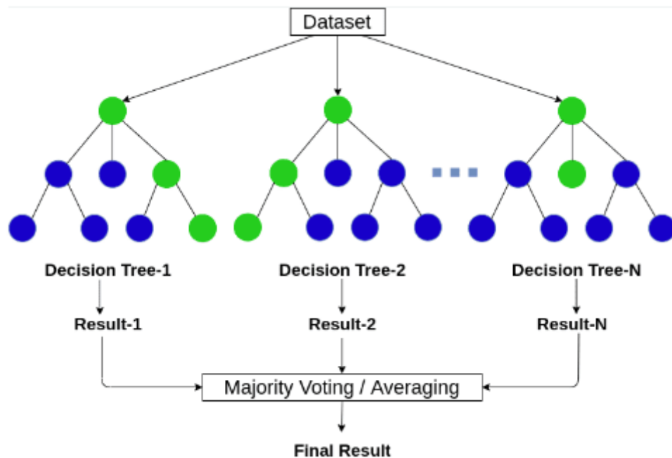
Hình 2.1 Sơ đồ nguyên lý hoạt động của thuật toán Random Forest
