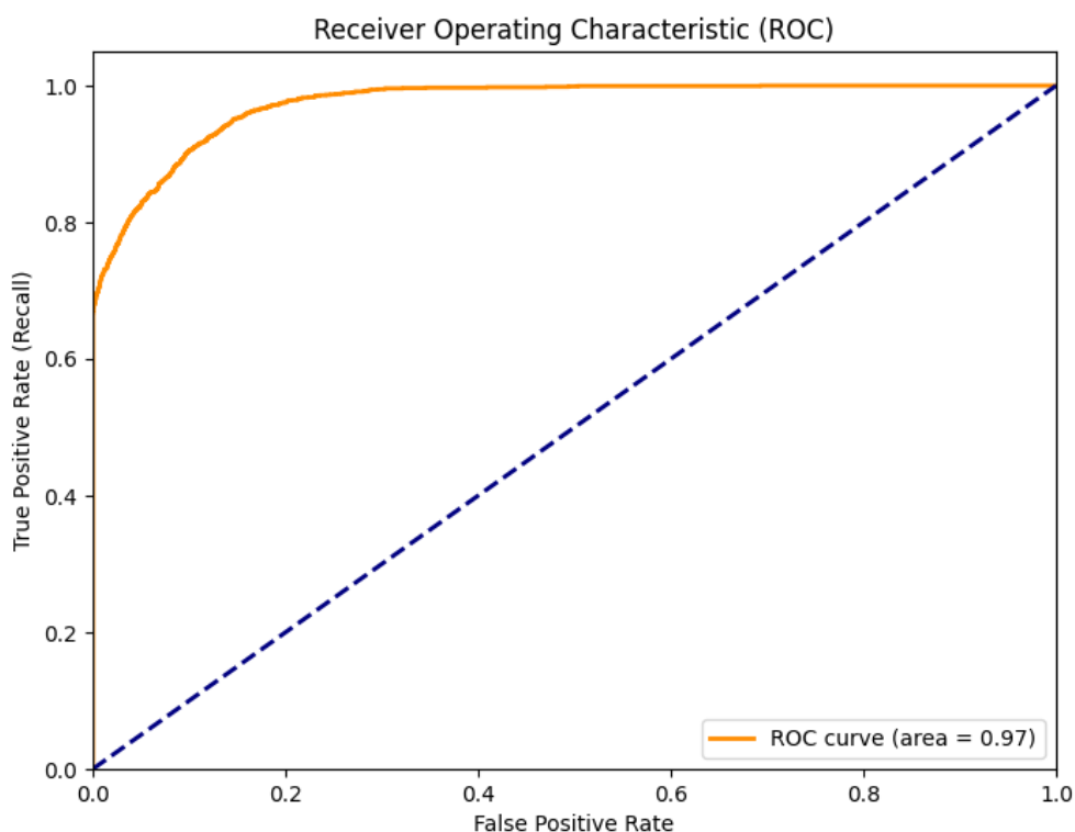
Hình 5.2 Biểu đồ ROC Curve
