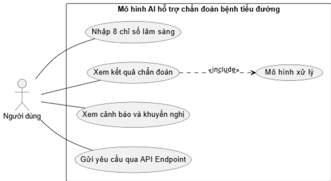
Hình 3.1 Sơ đồ use case mô hình AI hỗ trợ chẩn đoán bệnh tiểu đường
