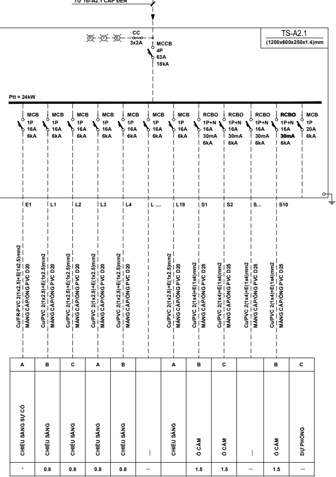
SƠ ĐỒ TỦ ĐIỆN CÔNG CỘNG XƯỞNG A2 KHU A
