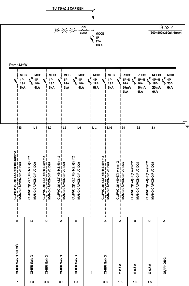
SƠ ĐỒ TỦ ĐIỆN CÔNG CỘNG XƯỜNG A2 KHU B
