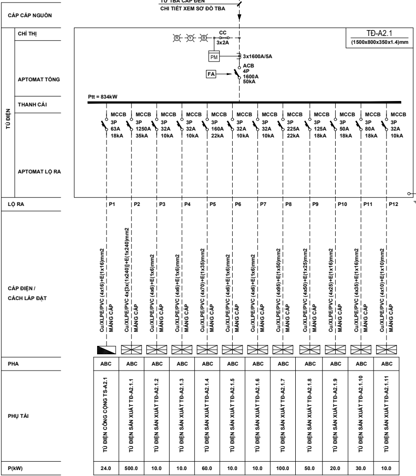
SƠ ĐỒ TỦ ĐIỆN TỔNG NHÀ XƯỞNG A2 KHU A
