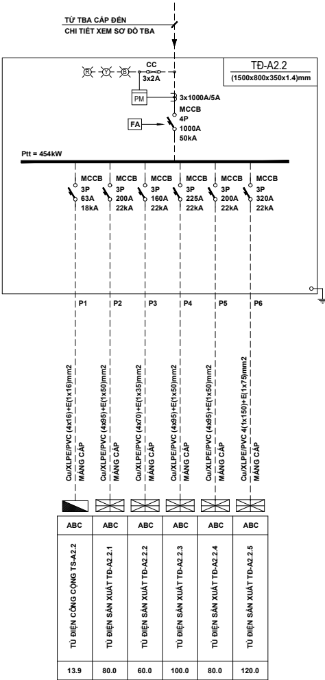
SƠ ĐỒ TỦ ĐIỆN TỔNG NHÀ XƯỜNG A2 KHU B
