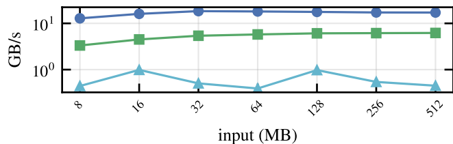
XML
