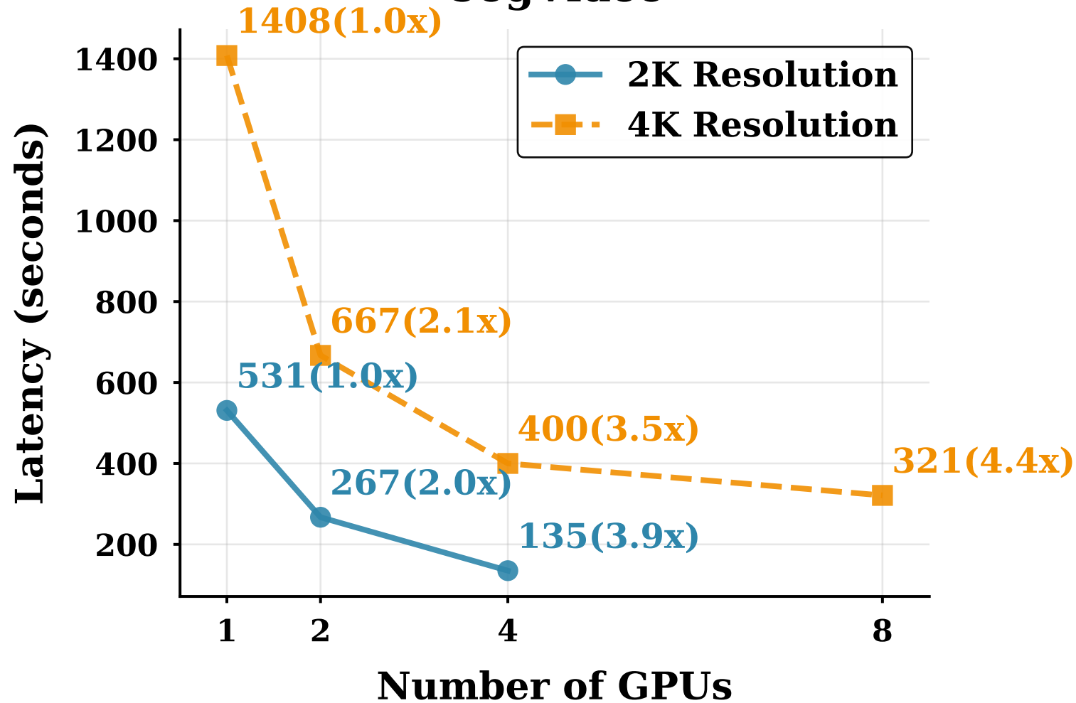
CogVideo
