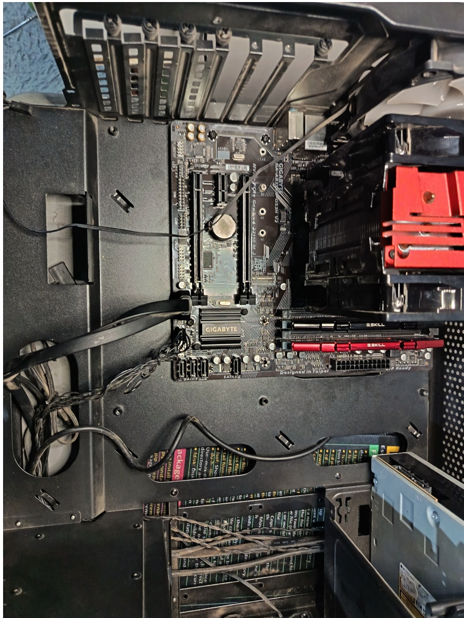
Figura 8. Primeros cables conectados a la tarjeta madre.
