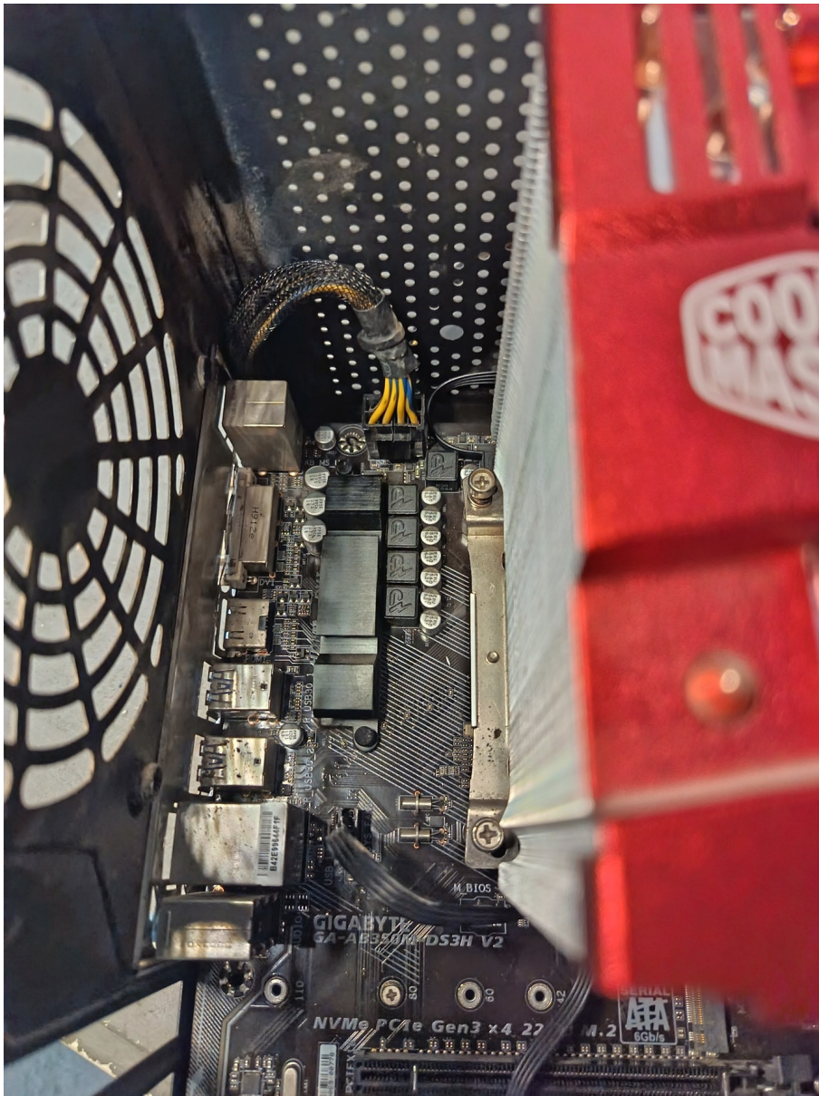
Figura 10. Cable de alimentación del procesador conectado a la placa.
