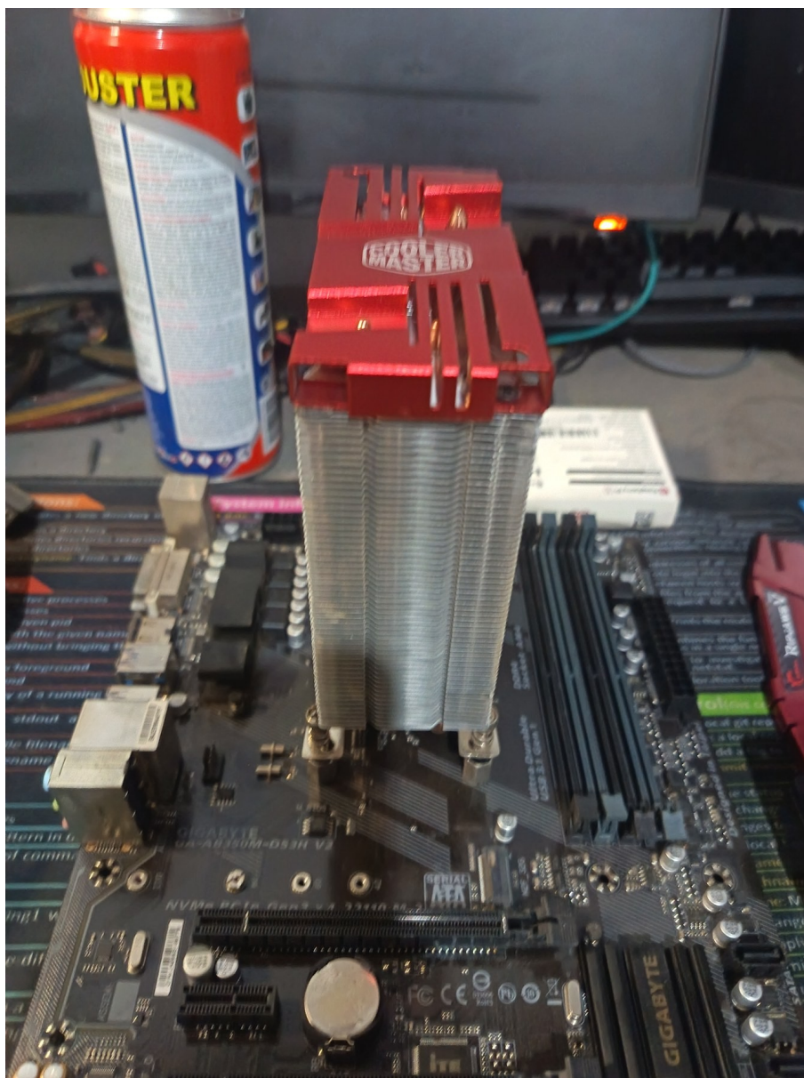
Figura 5. Cooler Master Hyper 212 Red sobre el socket AM4.
