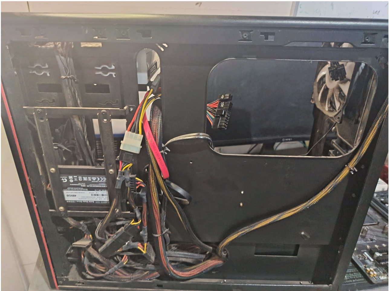
Figura 12. Cableado ordenado en el lado posterior de la bandeja.
