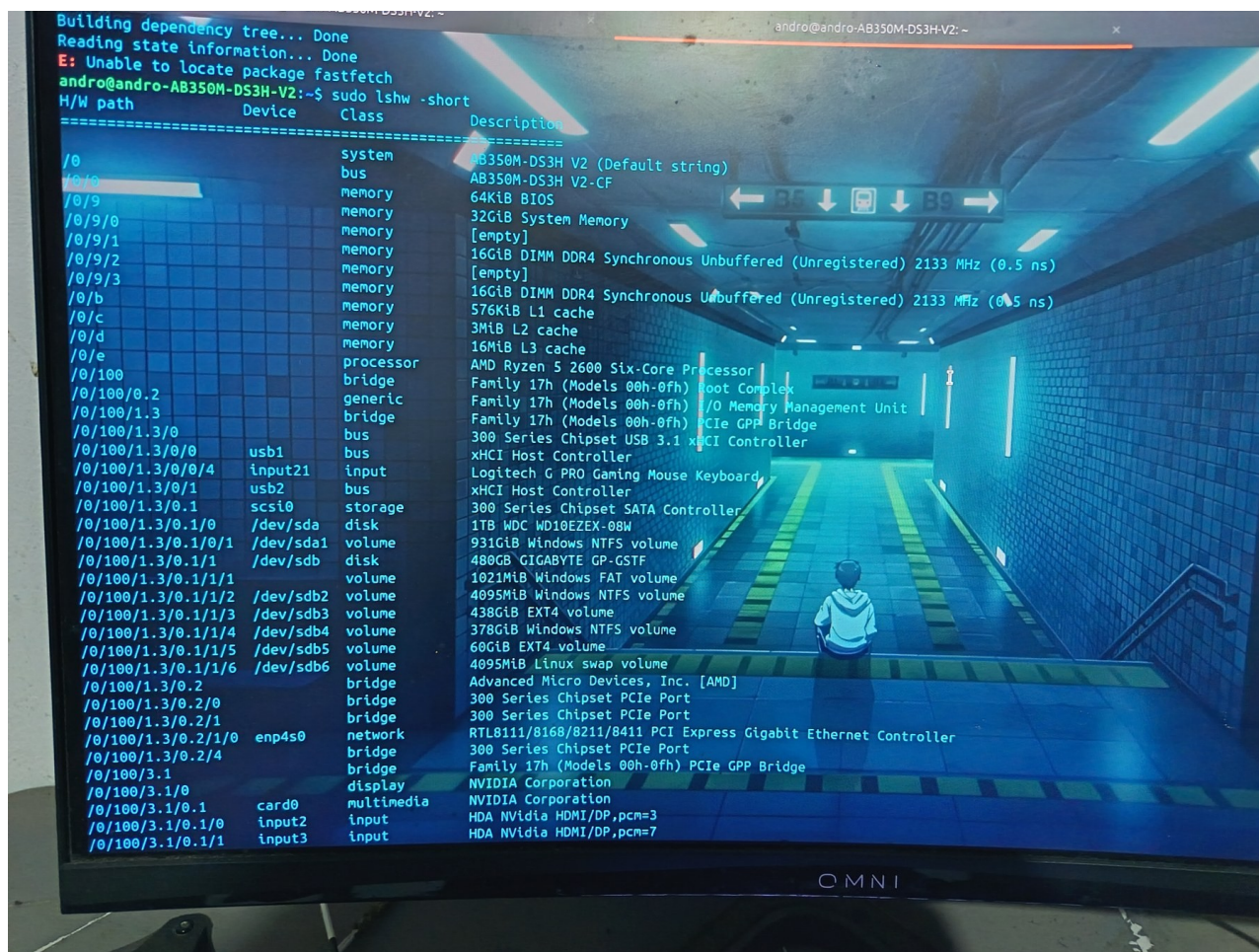
Figura 15. Salida del comando «sudo lshw -short» en el equipo.
