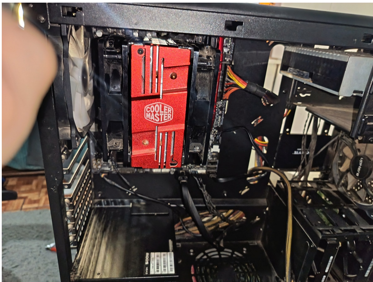
Figura 11. Conector principal y cables restantes conectados.
