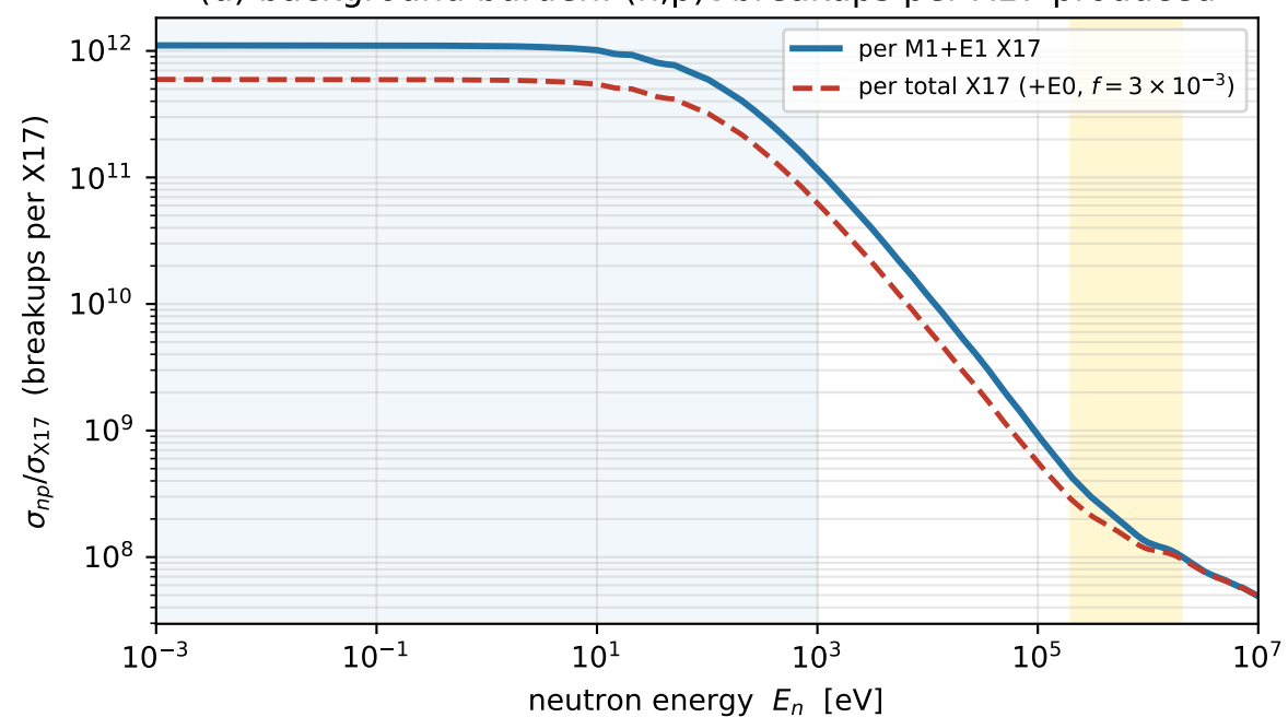
(d) background burden: (n,p)t breakups per X17 produced
