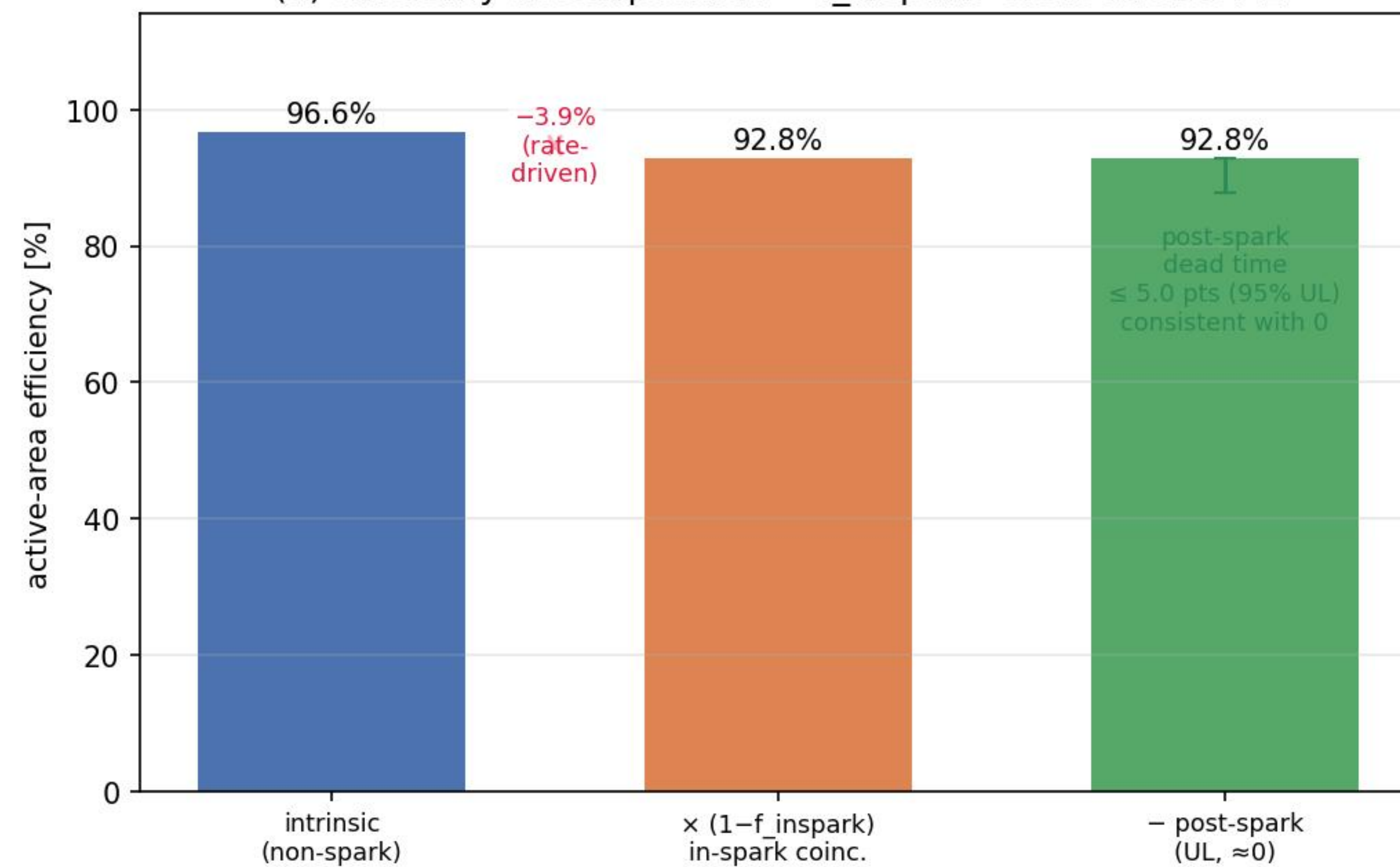
(d) efficiency decomposition — f_{\text{inspark}}=3.9\% at 0.33 Hz
