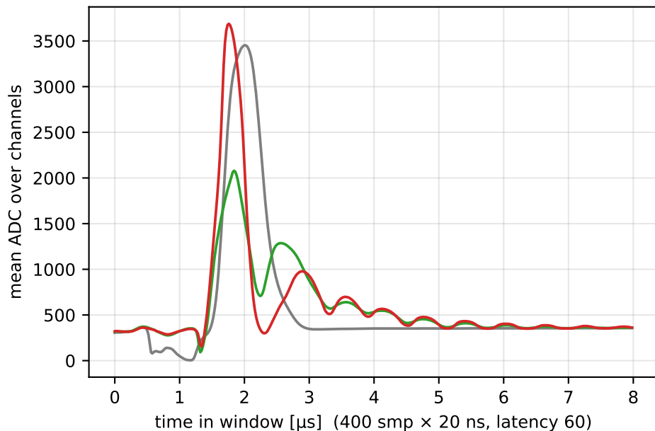
detector C (FEU 07, x-plane)
