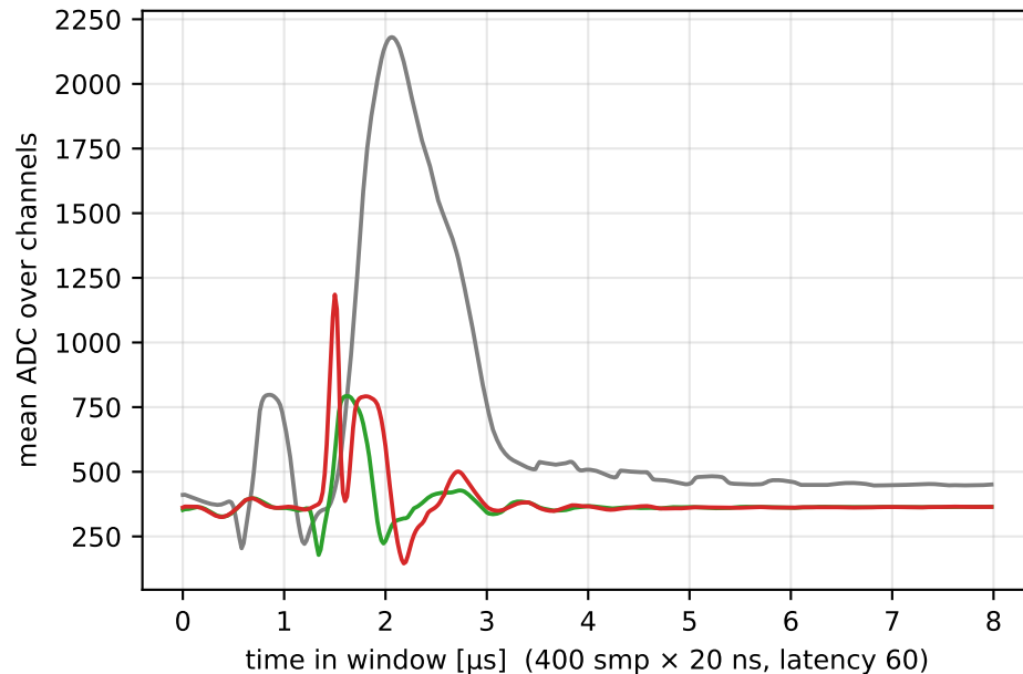
detector D (FEU 01, x-plane)
