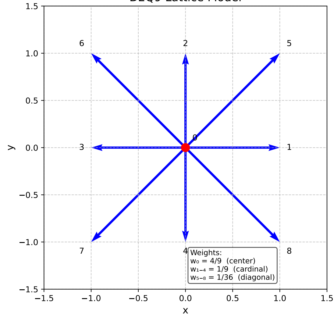
D2Q9 Lattice Model
