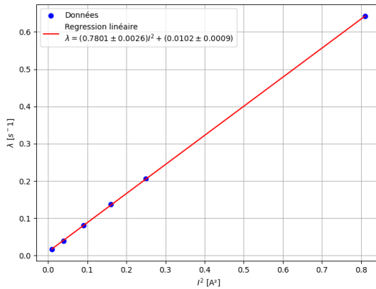
Figure 5: lambdas en fonction des courants
