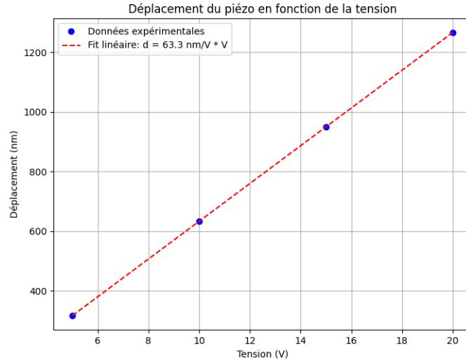
Figure 9: Courbe d(V) permettant de déterminer le coefficient piézoélectrique d_{33} . La pente de la droite correspond à la valeur expérimentale de d_{33} .
