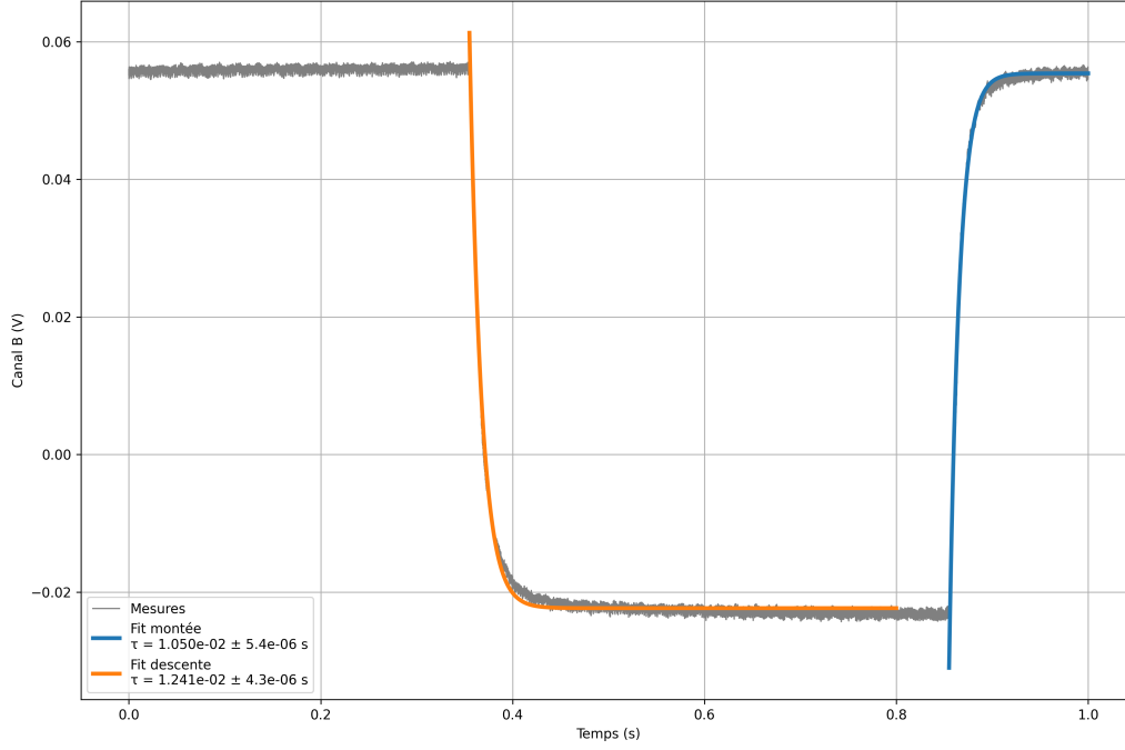
Figure 5: Courbe de fluage montrant la réponse temporelle du piézoélectrique à un saut de tension.
