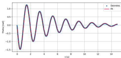
Figure 15: Mesure de l'angle theta a 0.5A
